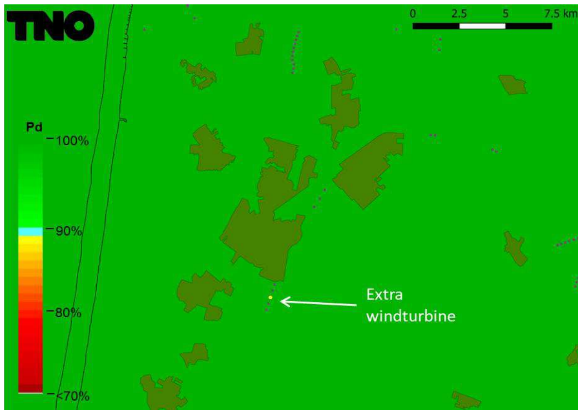
Figuur 8 Detectiekans van het primaire verkeersleidingsradarnetwerk op 1000 voet boven het bouwplan nadat deze is gerealiseerd. De locatie van de nieuwe windturbine is aangegeven met gele stip.
