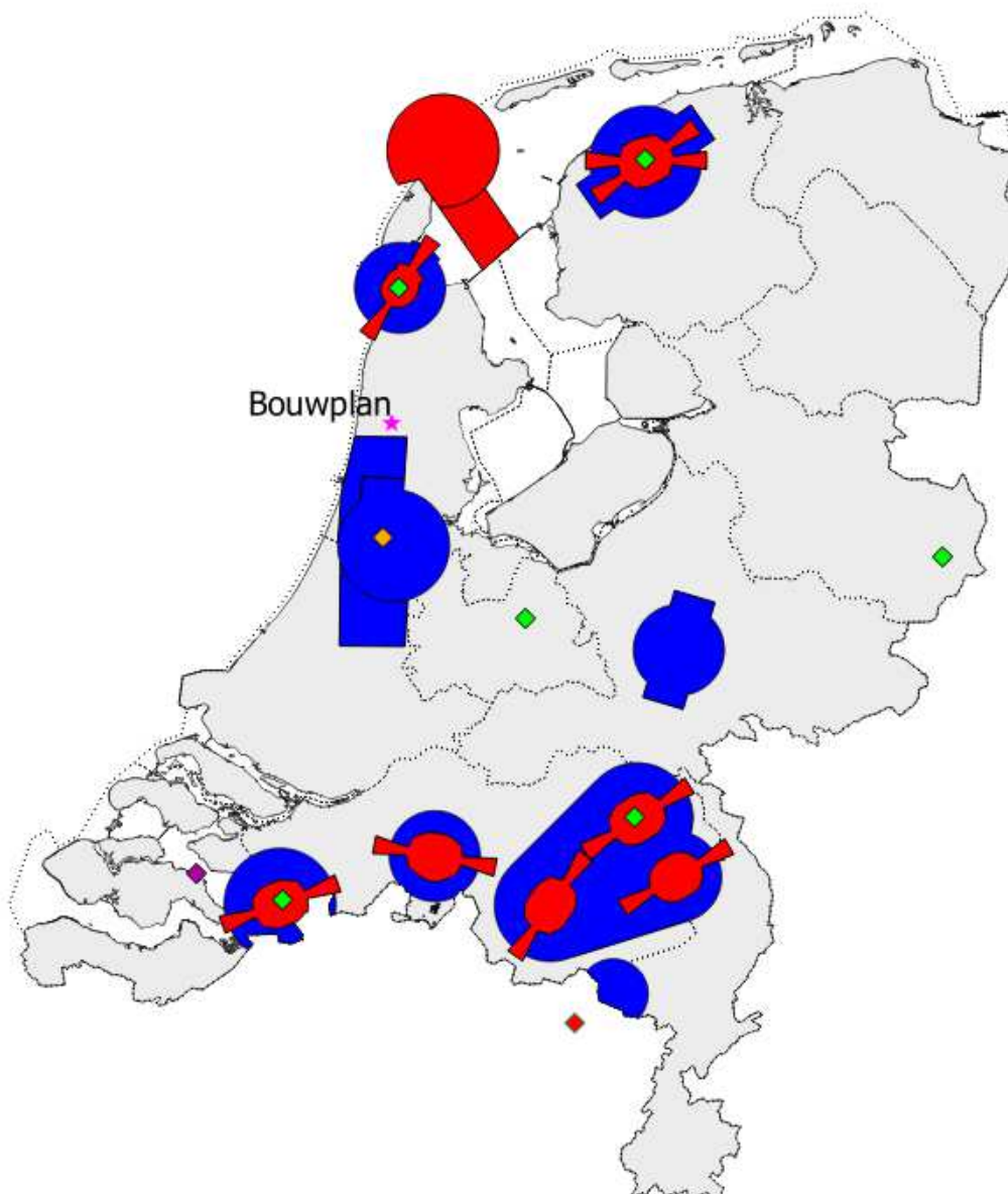
Figuur 6 De ligging van het te toetsen bouwplan aangegeven met een ster en de ligging van de thans gehanteerde 2023 normhoogtes op 300 voet (rood) en 500 voet (blauw). Op 1000 voet (paars) dient het verkeersleidingsradarnetwerk,
