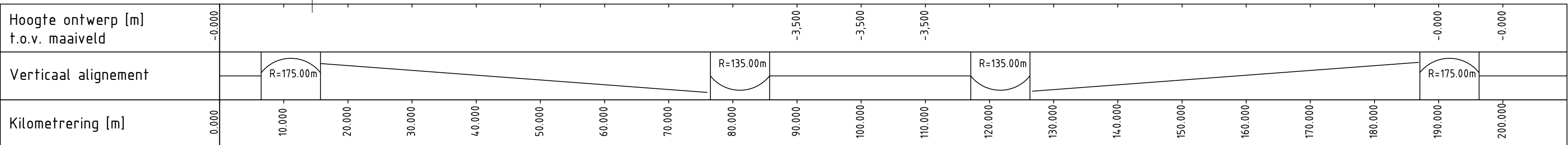
Principe lengteprofiel: Fietstunnel Vert. schaal 1:100 Hor. schaal 1:500
