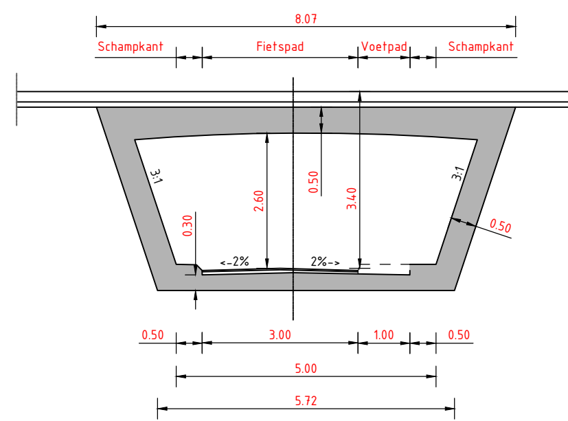
Principe profiel fietstunnel Schaal 1:100
