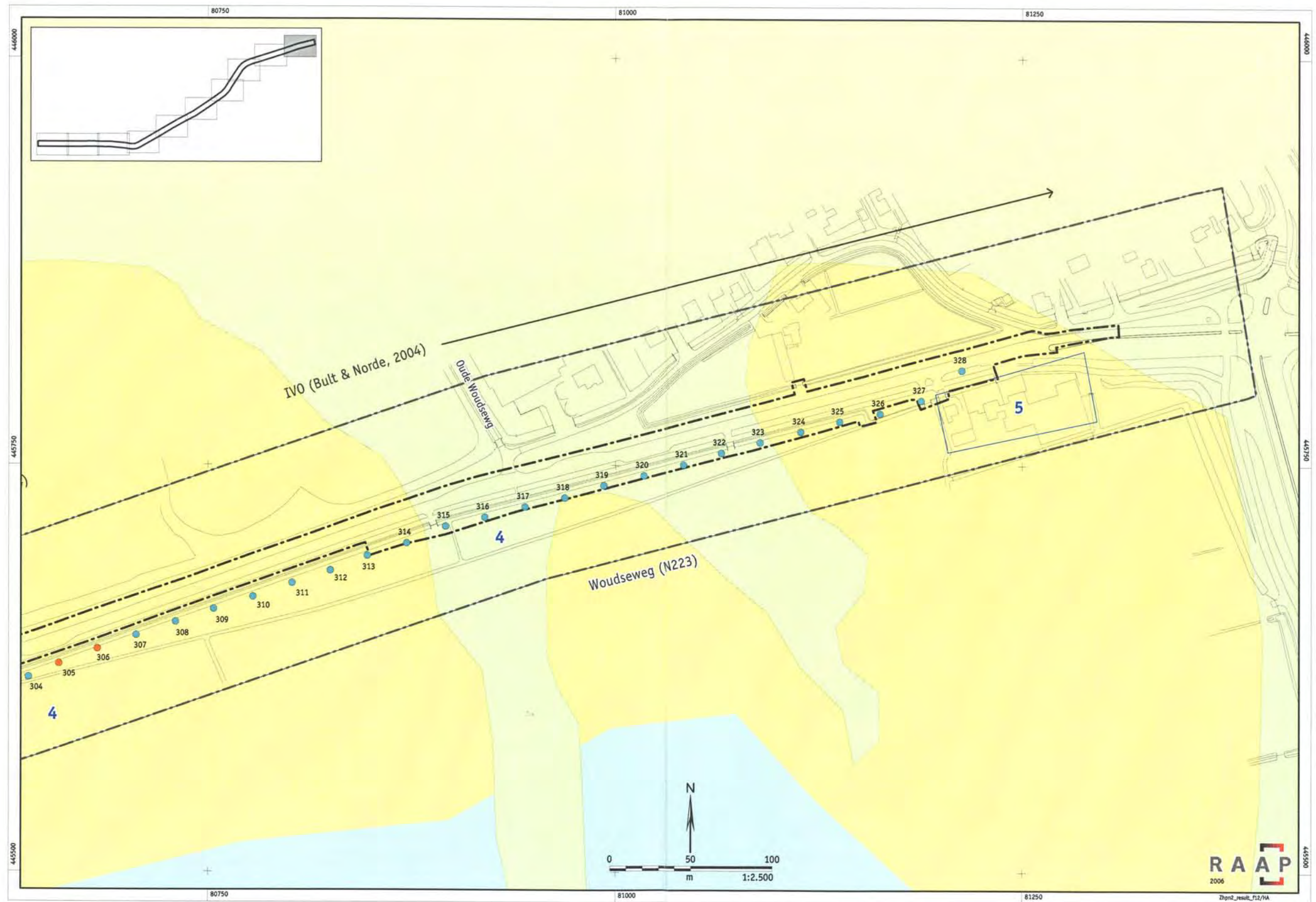
Bijlage 1. Resultaten booronderzoek - Blad 10.
