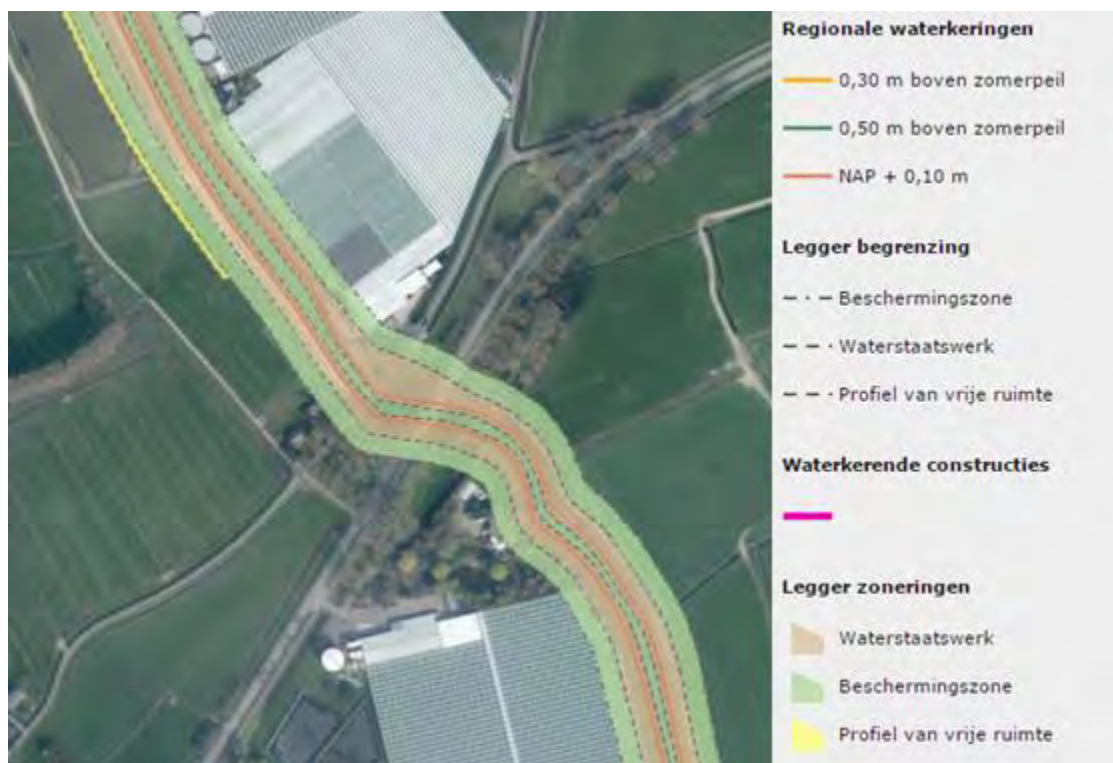
Afbeelding 37: Uitsnede legger Regionale waterkering (bron: legger Hoogheemraadschap van Delfland)
