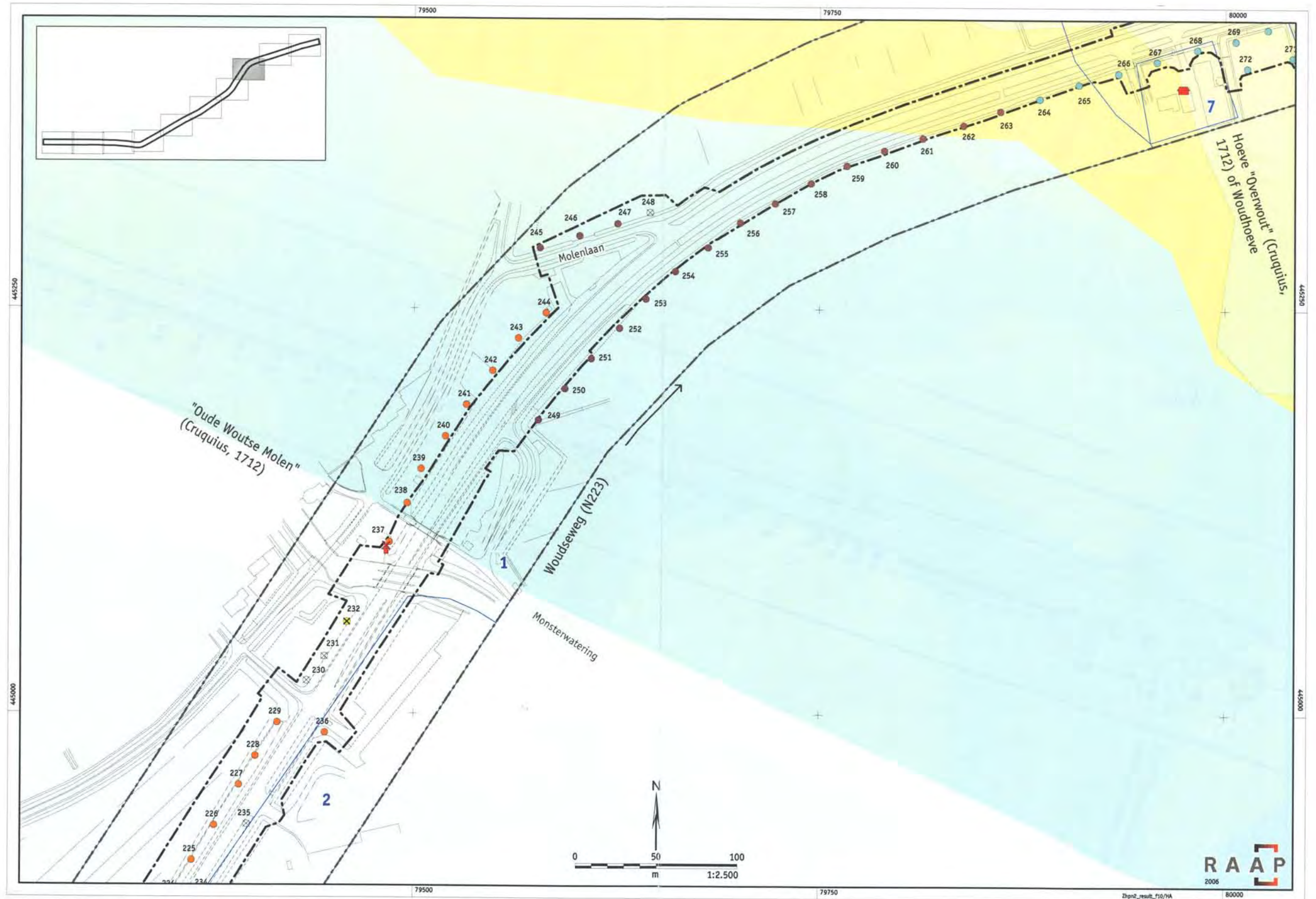
Bijlage 1. Resultaten booronderzoek - Blad 8.
