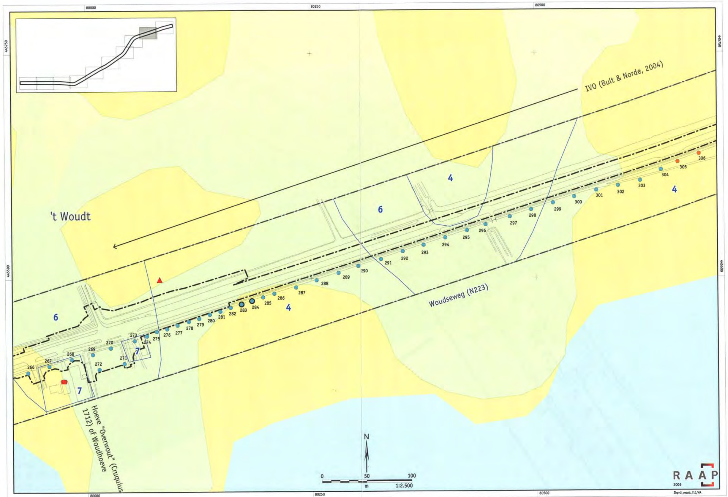
Bijlage 1. Resultaten booronderzoek - Blad 9.
