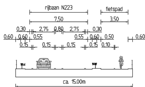
Figuur 26: Profiel R-A, profiel brug
