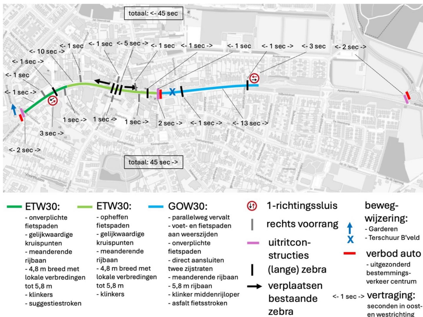
Figuur 6: Maatregelen ETW30 Hoofdstraat inclusief geschatte tijdvertraging
