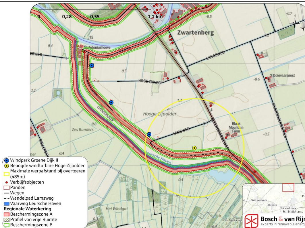
Figuur 2 Aanwezigheid van voor externe veiligheid relevante onderwerpen binnen de invloedssfeer van de windturbine (de maximale werpafstand bij overtoeren).
