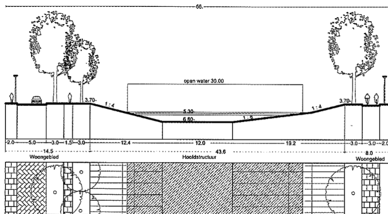
W1b 30m open water - Standaard + duurzame oevers
