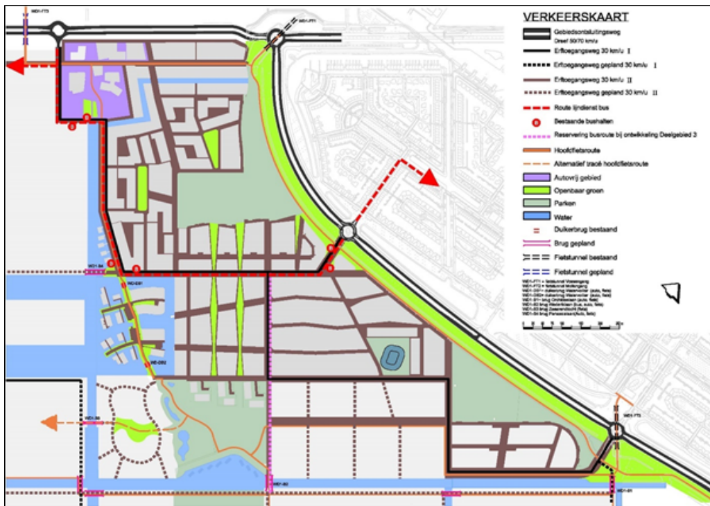
Afbeelding 3: Ontsluitingsstructuur Warande Deelgebied 1 (afkomstig uit Toolbox Warande) en rood omkaderd woningbouw Klein Nooten.
