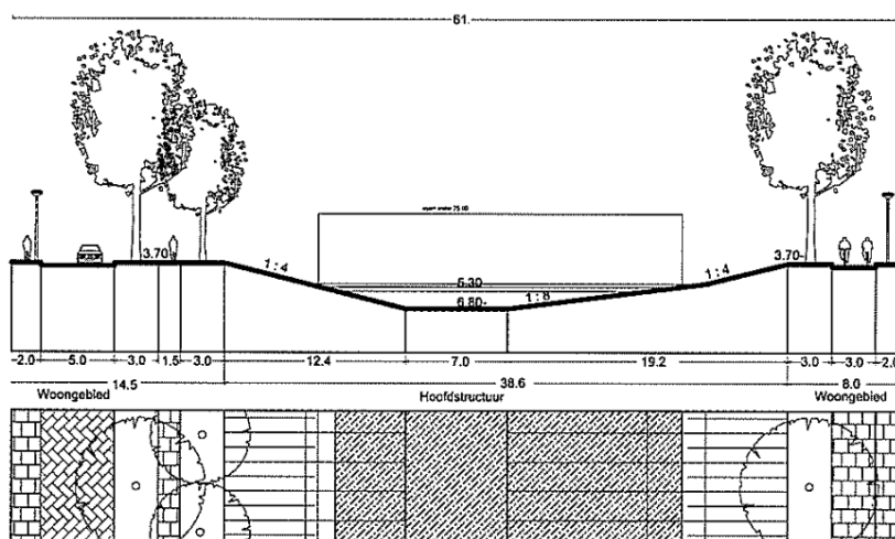
W2b 25m open water - standaard + duurzame oevers
