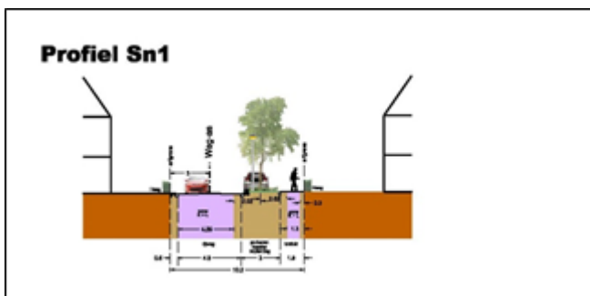
Afbeelding 5: Dwarsprofiel van standaard woonstraat (Sn1), met ruimte voor plantvakken met kleine bomen aan één zijde van de straat.
