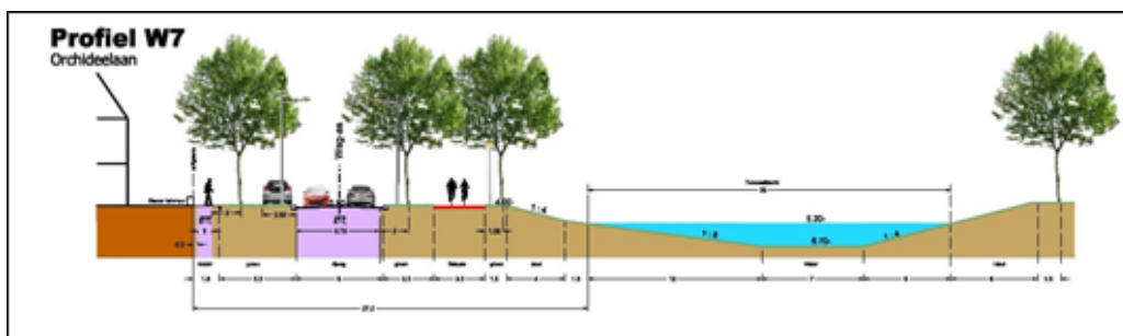
Afbeelding 4: Dwarsprofiel van gebiedsontsluiting Orchideelaan (W7), met begeleidende bomenrij en vrijliggend fietspad.
