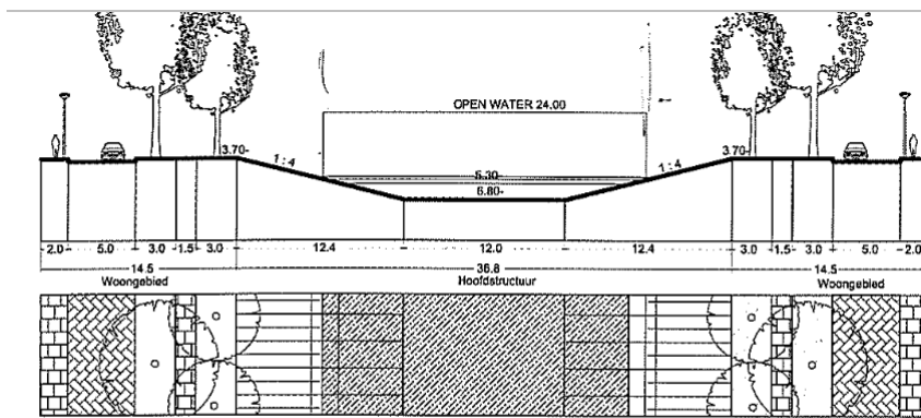
W1: 24 m open water - standaard oever:
