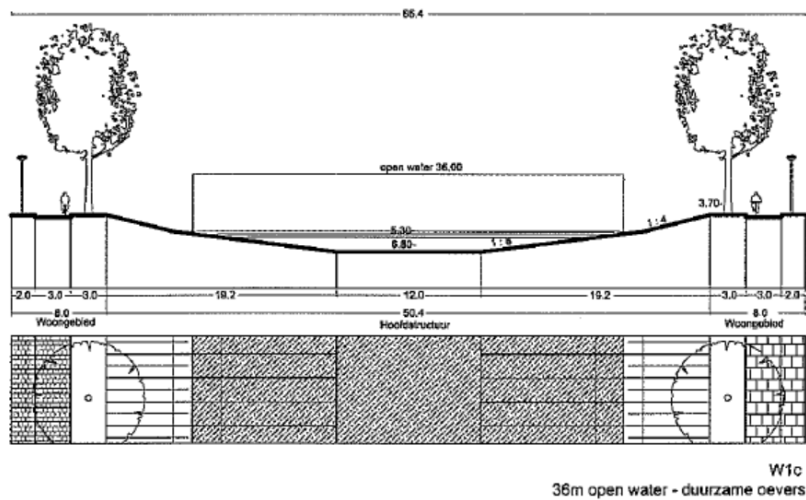
Afbeelding 1: Uitgangspunten inrichting oevers
