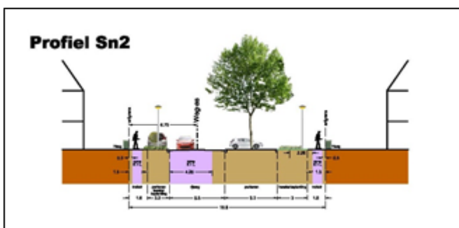
Afbeelding 6: Dwarsprofiel van de brede woonstraat (Sn2) met in het midden ruimte voor een groenstrook met grote bomen en daartussen haaks parkeren.
