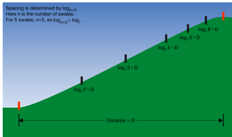
Figuur 3. Logaritmische verdeling van de afstand tussen swales op een hellend perceel, naar Barnes (2015).
