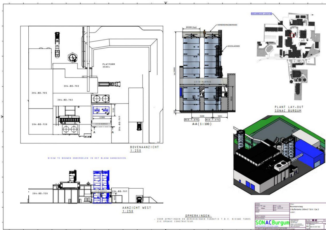
figuur 3: ligging tanks cat. 2 fabriek
