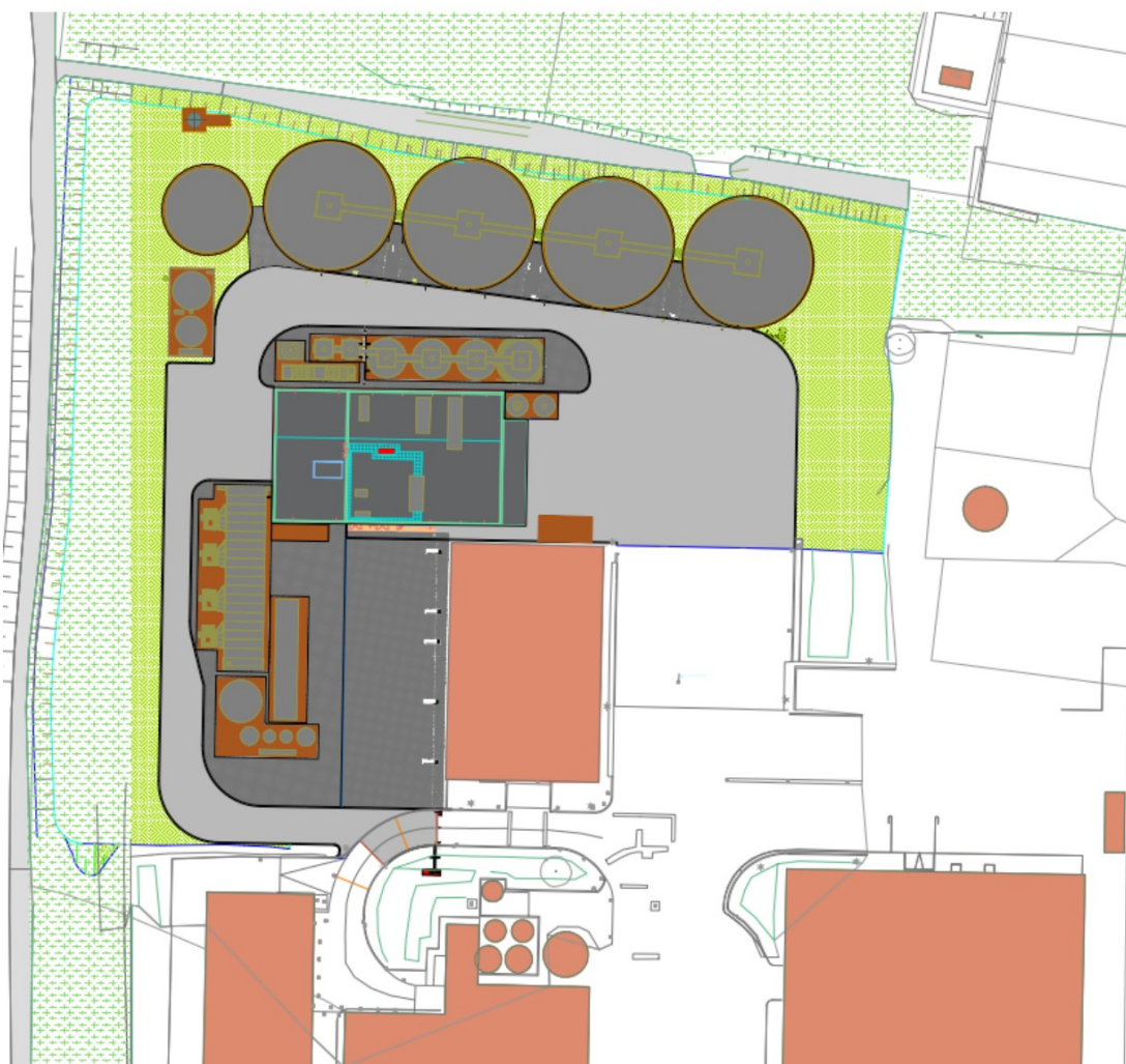
figuur 2: plattegrond terrein project 'Groen Gas'
