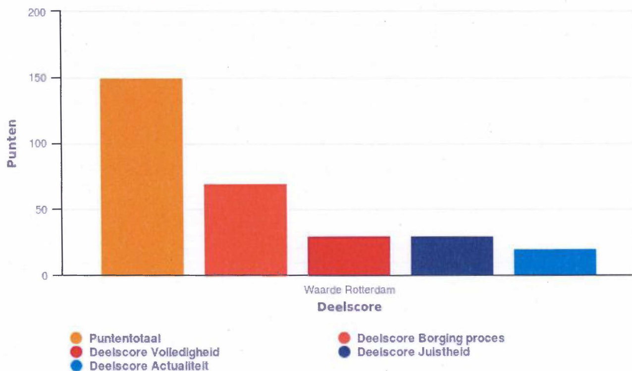
BGT 2.1 Overzichtsdigram
