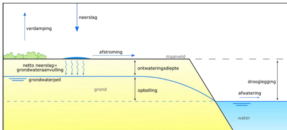
Figuur 8. Schematisatie van enkele hydrologische begrippen.
