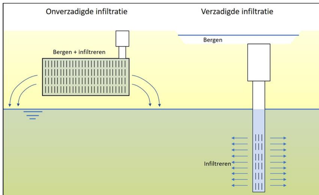
Figuur 12. Schematische weergave verschillende methodes voor de toepassing van infiltratie. Links op kleine diepte (bijvoorbeeld waterbergende wegfundering of infiltratiekratten, waar nodig gecombineerd met drainage). Rechts op grotere diepte (bijvoorbeeld met een IT-riool, of diepte-infiltratie met urban water buffer), eventueel gecombineerd met berging aan maaiveld.
