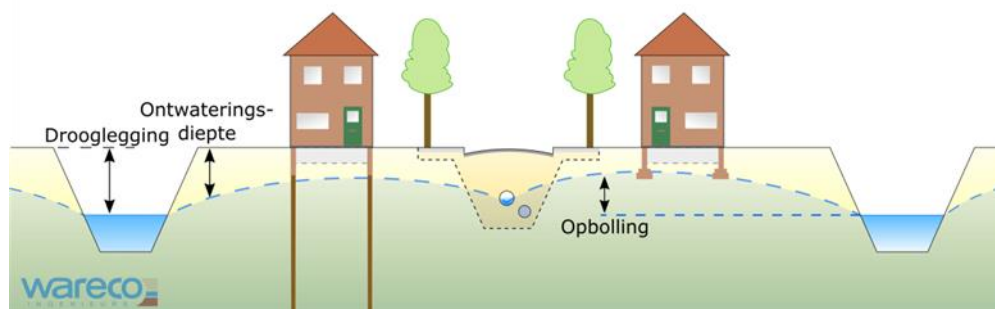
Figuur 13. Voorbeeld van het verloop van de grondwaterstand bij openbaar terrein ten opzichte van particuliere percelen, in zandige gebieden.
