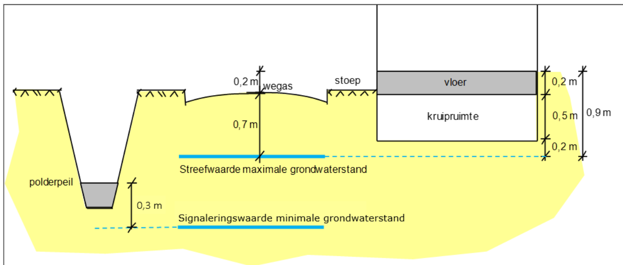
Figuur 10. Streefwaarde voor maximale grondwaterstanden beneden het straatpeil ten opzichte van de kruipruimte en signaleringswaarde voor de minimale grondwaterstand beneden het oppervlaktewaterpeil, in bestaand bebouwd gebied met veenlagen (met een gangbaar profiel van de openbare weg ten opzichte van de woninghoogte).
