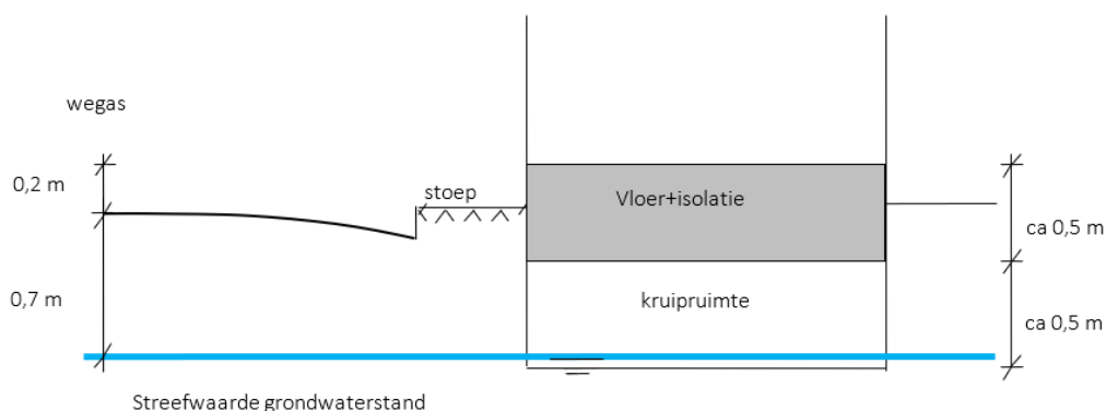
Figuur 11. Schematische weergave streefwaarde grondwaterstand onder kruipruimtebodembodem bij nieuwbouwwoningen met dikke constructievloeren.
