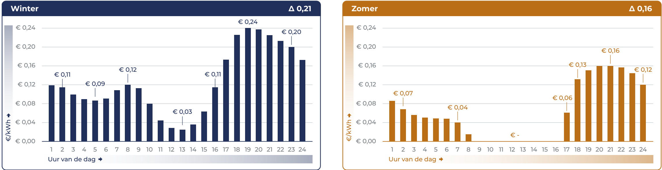
Figuur 1 Uurtarieven voor een nieuw tariefstelsel, zoals gehanteerd voor de doorrekeningen in dit onderzoek 9) . Links het tarief voor de ‘winter’-periode (oktober – april) en rechts de ‘zomer’ (april – oktober). Zie voor toelichting op het transporttarief figuur 4 . Dit betreft alleen afnametarieven, voorsnog is er geen invoedingstarief veronderstelt.
