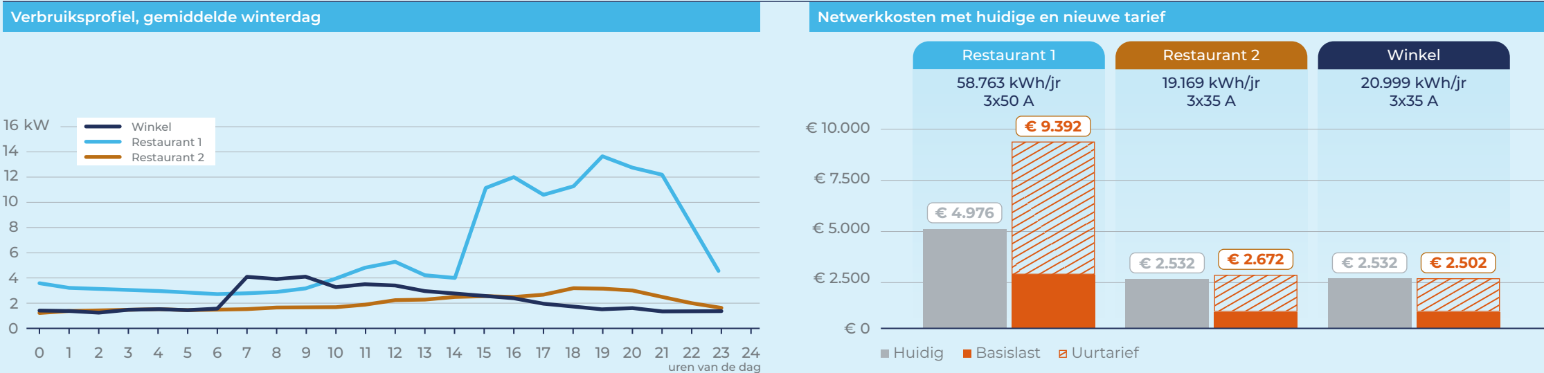
Figuur 25 Drietal verbruiksprofielen en netwerkkosten in 2030 van werkelijke profielen. Data beschikbaar gesteld door COMCAM (Restaurant 1 & 2) en Scholt Energy (Winkel).
