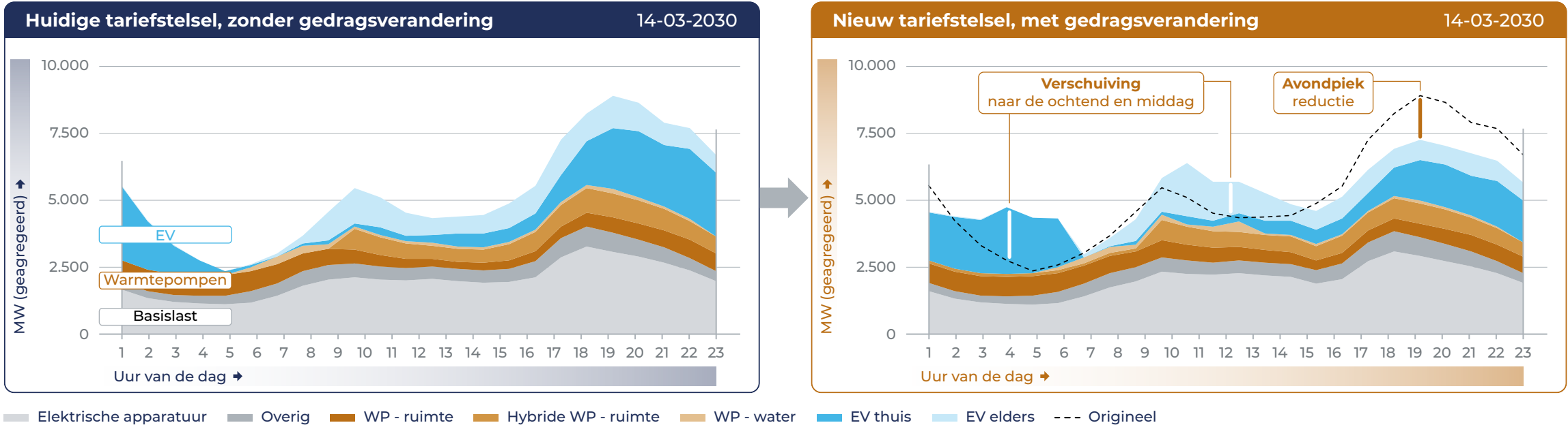
Figuur 2 Voorbeeld van vraagverschuiving door tariefstelwijziging. Grafieken lichten het geaggregeerde profiel van alle woningen in Nederland op één dag uit in 2030. 10) De blauwe vlakken vertegenwoordigen elektrische voertuigen (EV), de bruine (hybride) warmtepompen en de grijze de overige elektrische apparatuur.
