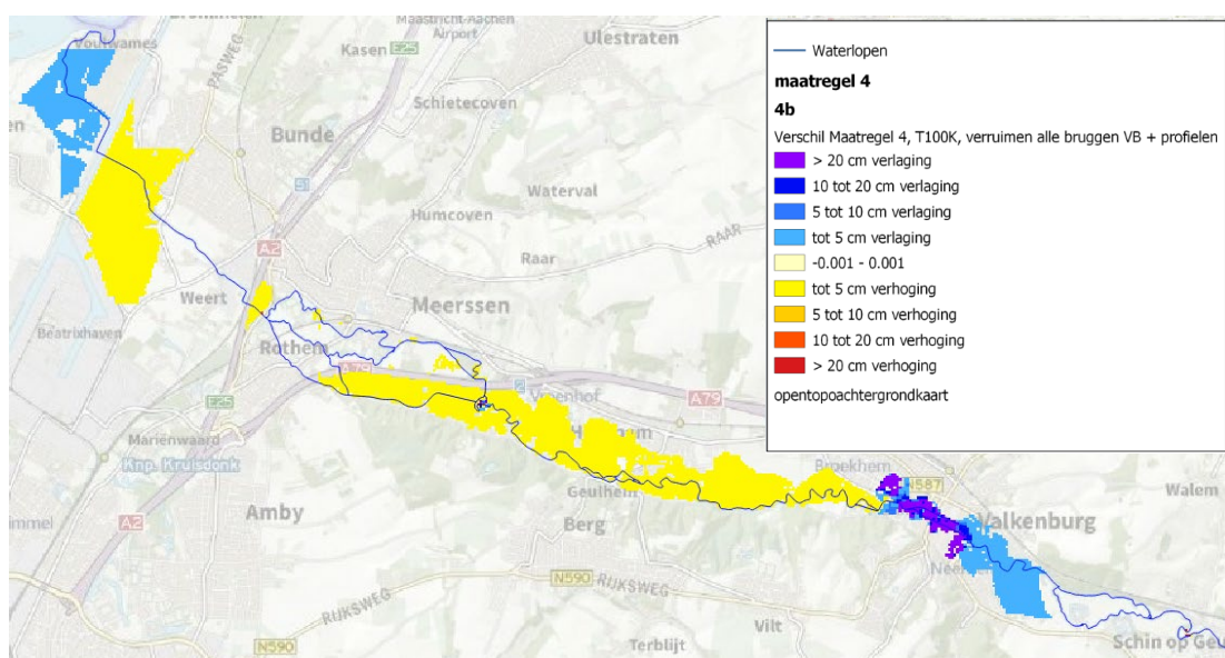
Figuur 5.15 Waterstandsverandering als gevolg van het veruimen van bruggen en duikers en het verdubbelen van de afvoercapaciteit bij Valkenburg voor juli 2021 (verschil max. waterdiepte tussen referentie en maatregel, ingezoomd op de regio tussen Bunde en Valkenburg)
