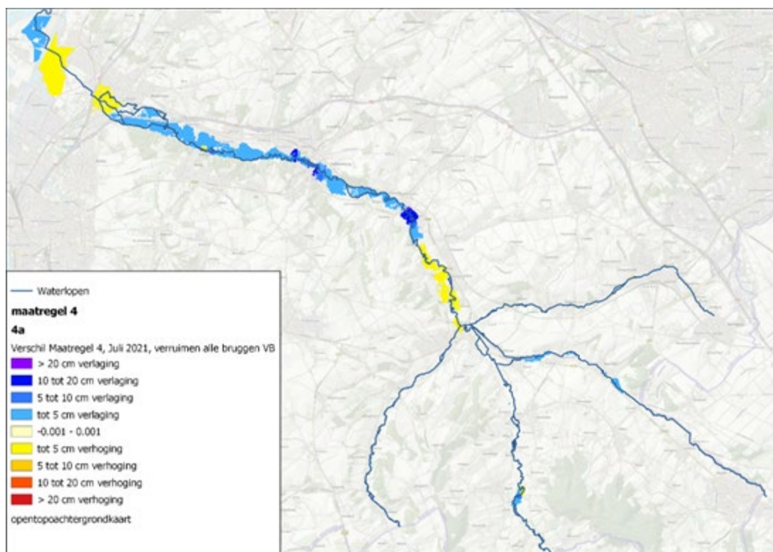
Figuur 5.14 Waterstandsverandering door het veruimen van duikers en bruggen voor juli 2021
