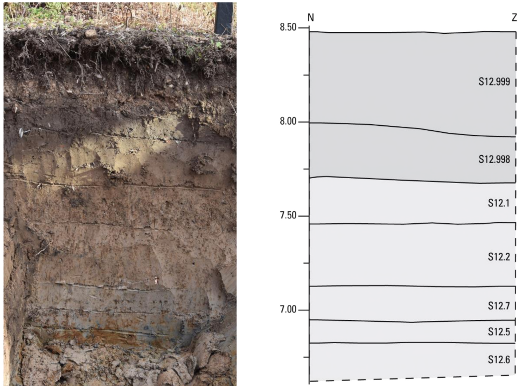
Fig. 5.1. Beuningen – De Asdonck. Profiel 12.1 met de oeverafzettingen op zand (S12.6).
