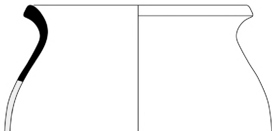
Fig. 7.3. Beuningen-De Asdonck. Een typisch Elmpt-randje van een bg-kog-2 of een bg-pot-2. Schaal 1:3.
