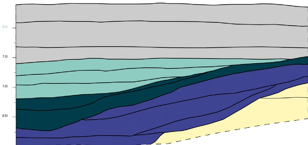
Fig. 6.2. Beuningen-De Asdonck. De grachtinsteek in het noordprofiel van werkput 7. Grijs: recente ophogingslagen en begraven bouwvoor; geel: natuurlijke lagen; paars: grachtfase 1; donkerblauw: grachtfase 2; lichtblauw grachtfase 3.
