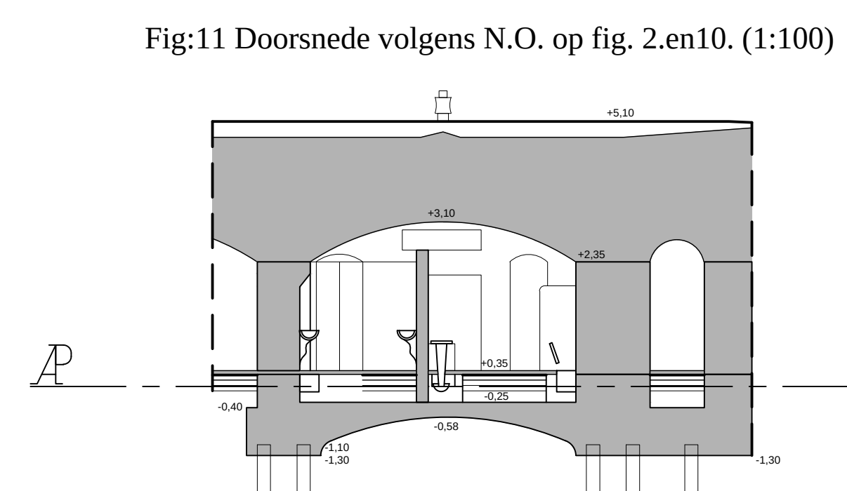
Fig:11 Doorsnede volgens N.O. op fig. 2.en10. (1:100)
