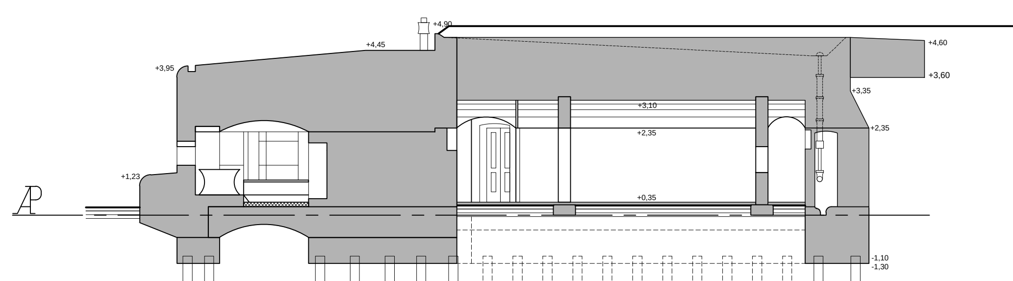
Fig:7 Doorsnede volgens G.H. op fig. 1.en 2. (1:100)
