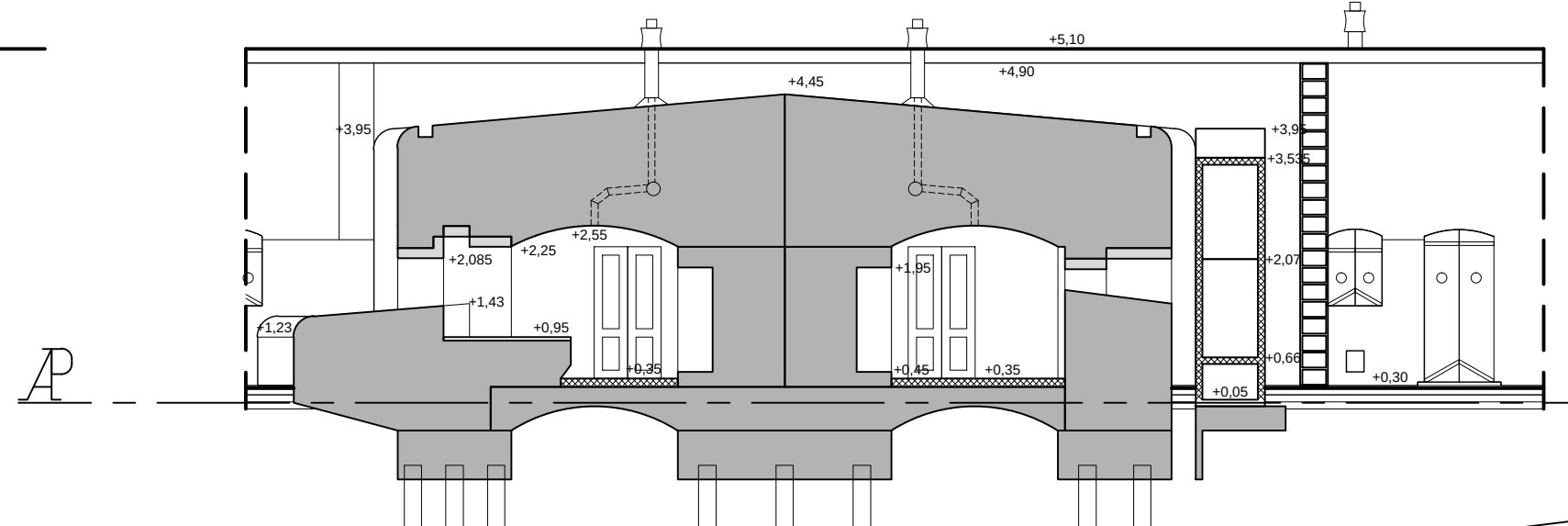
Fig:9 Doorsnede en standgezicht volgens L.M. op fig. 1.en 2. (1:100)
