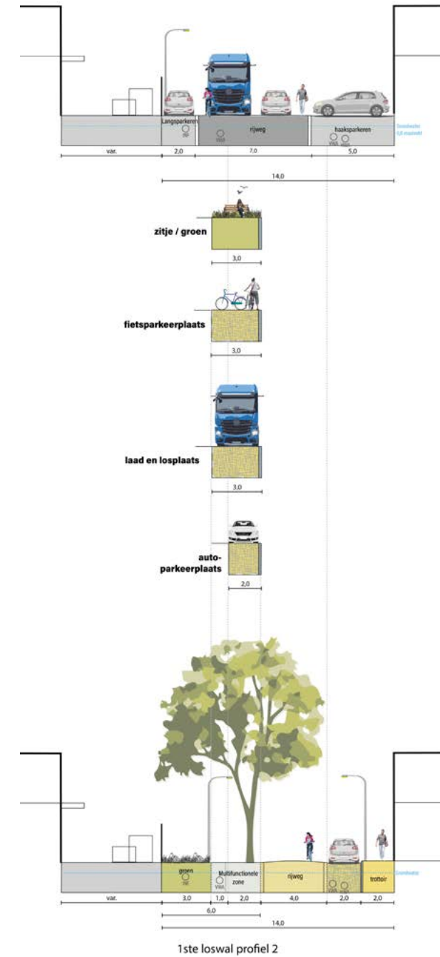
figuur II + III Dwarsdoorsnede en profiel 1e Loswal.
