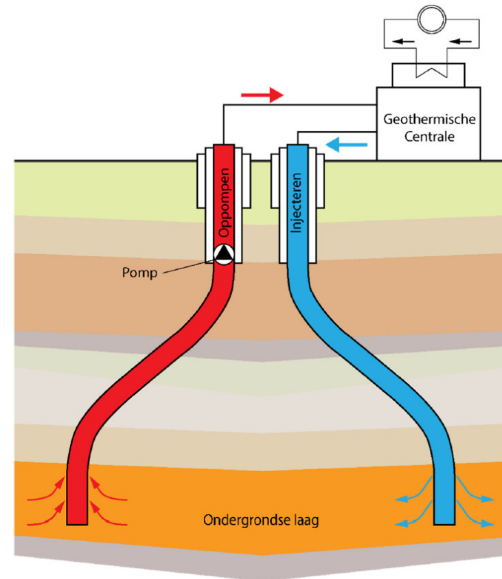
Figuur 14: Principe open bodemsysteem. Bron: taiboommilieu.be , 2024
