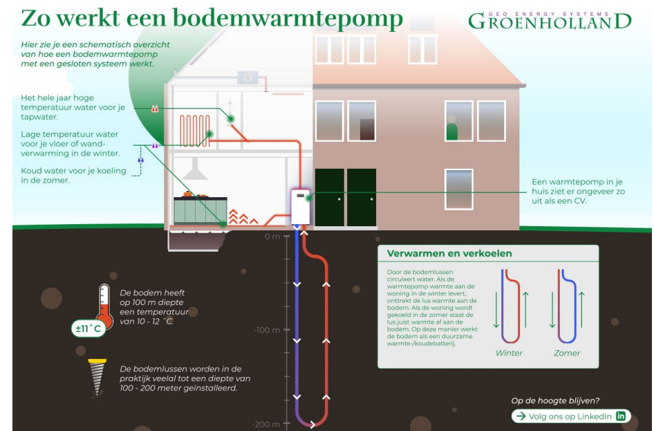
Figuur 15: Werking bodemwarmtepomp. Bron: GeoEnergyHolland, 2024
