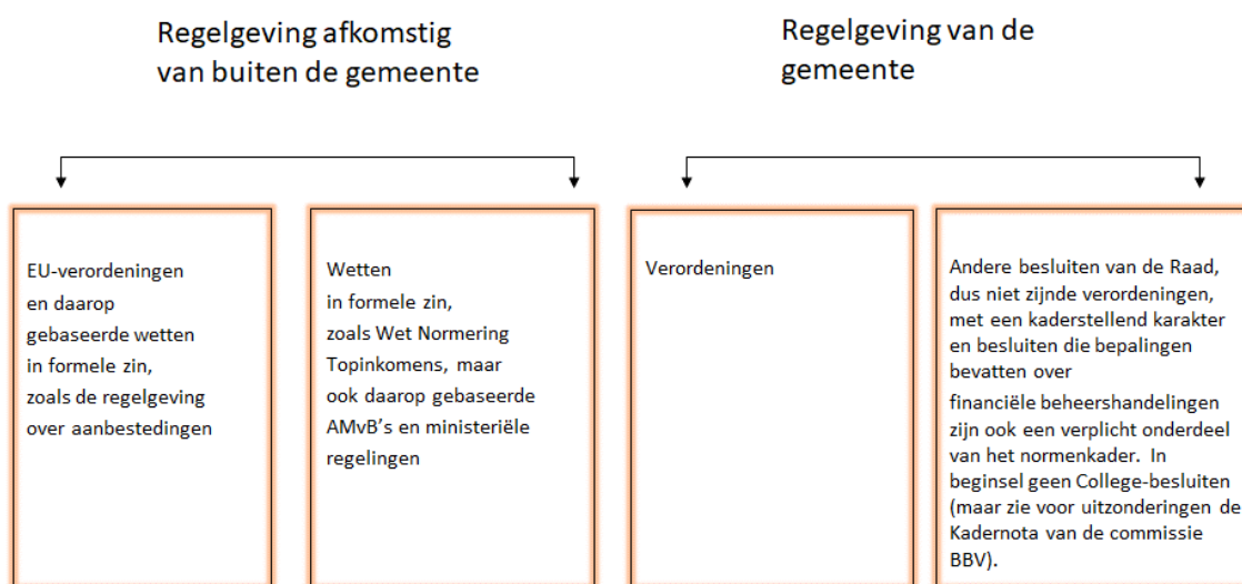
Figuur 4.1: Normenkader
