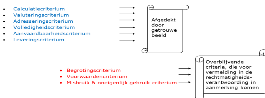
Figuur 4.2: Rechtmatigheidscriteria
