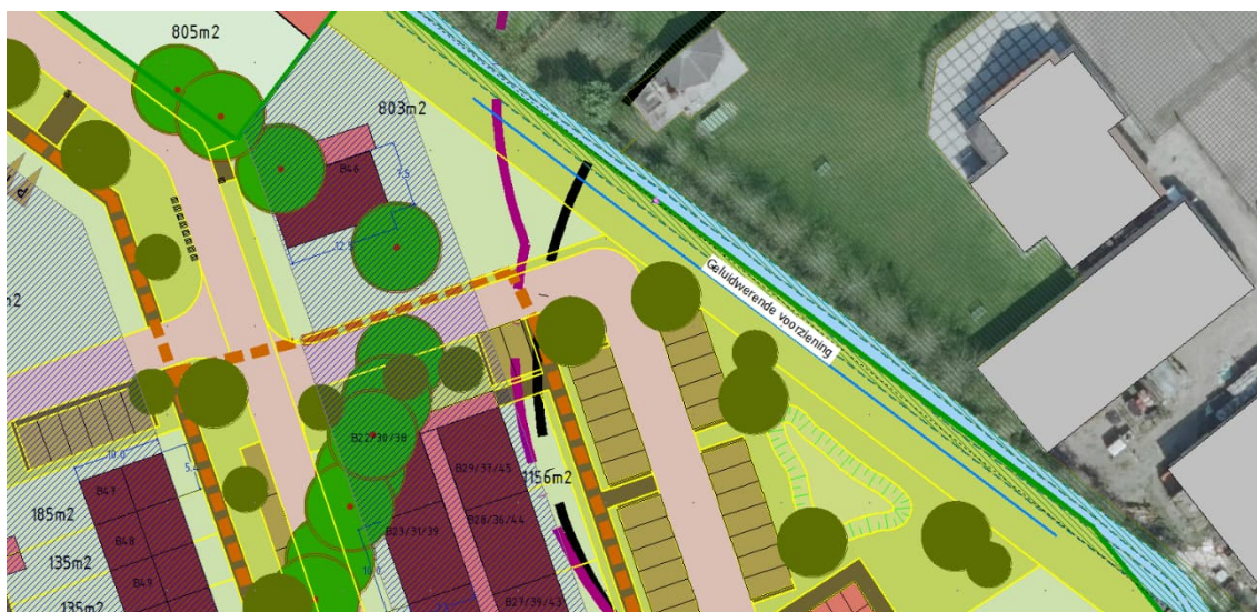
Afbeelding 8 Positie geluidwerende voorziening [blauwe lijn]
