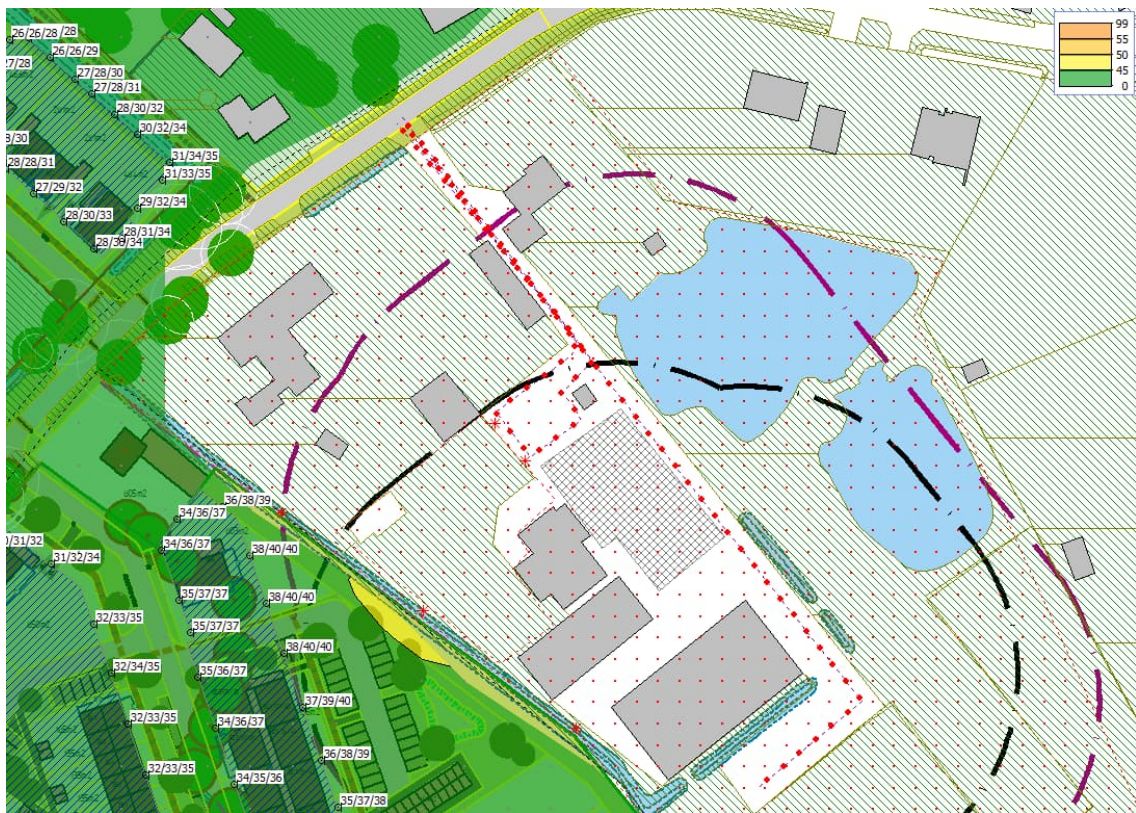
Afbeelding 7 Geluidsniveaus (etmaalwaarden) Hommelsedijk 6a
