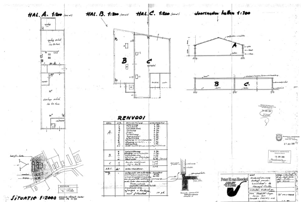
Afbeelding 4 Inrichtingstekening 'Hinderwetaanvraag bedrijfspanden Zandstraat 1 te Heeswijk-Dinther' d.d. 13-6-2006
