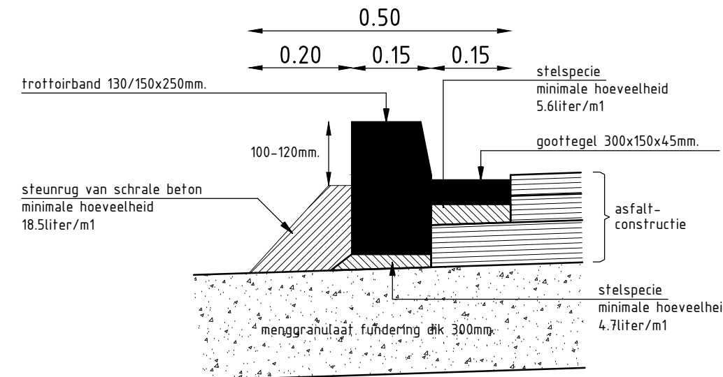
DOORSNEDE KANTOPSLUITING ASFALT met trotoirband 130/150x250mm.
