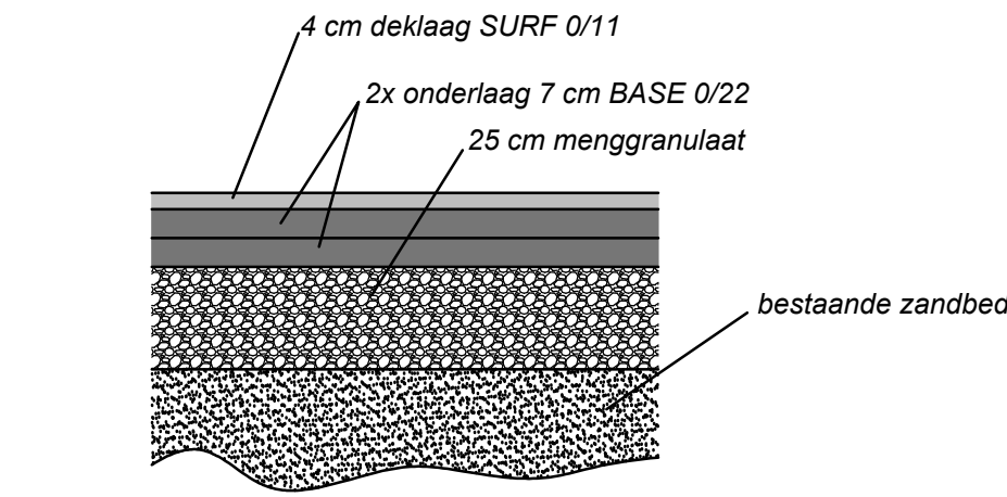
principe doorsnede laagopbouw nieuw asfalt
