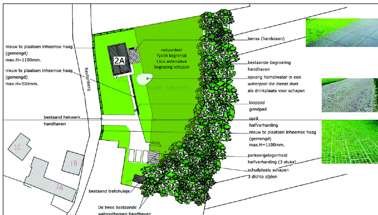
Situatietekening bouwplan
