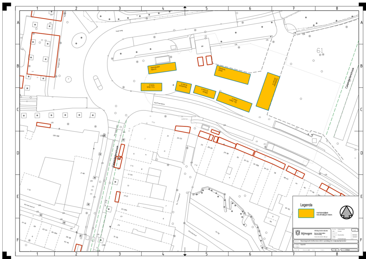
Tekening warenmarkt Kelfkensbos (maandag) 1
