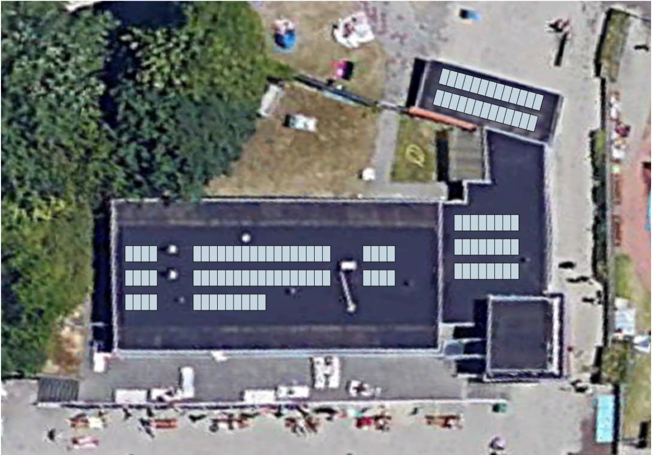
Afbeelding 6, Dakoverzicht Goffertbad met mogelijke zonnepanelen
