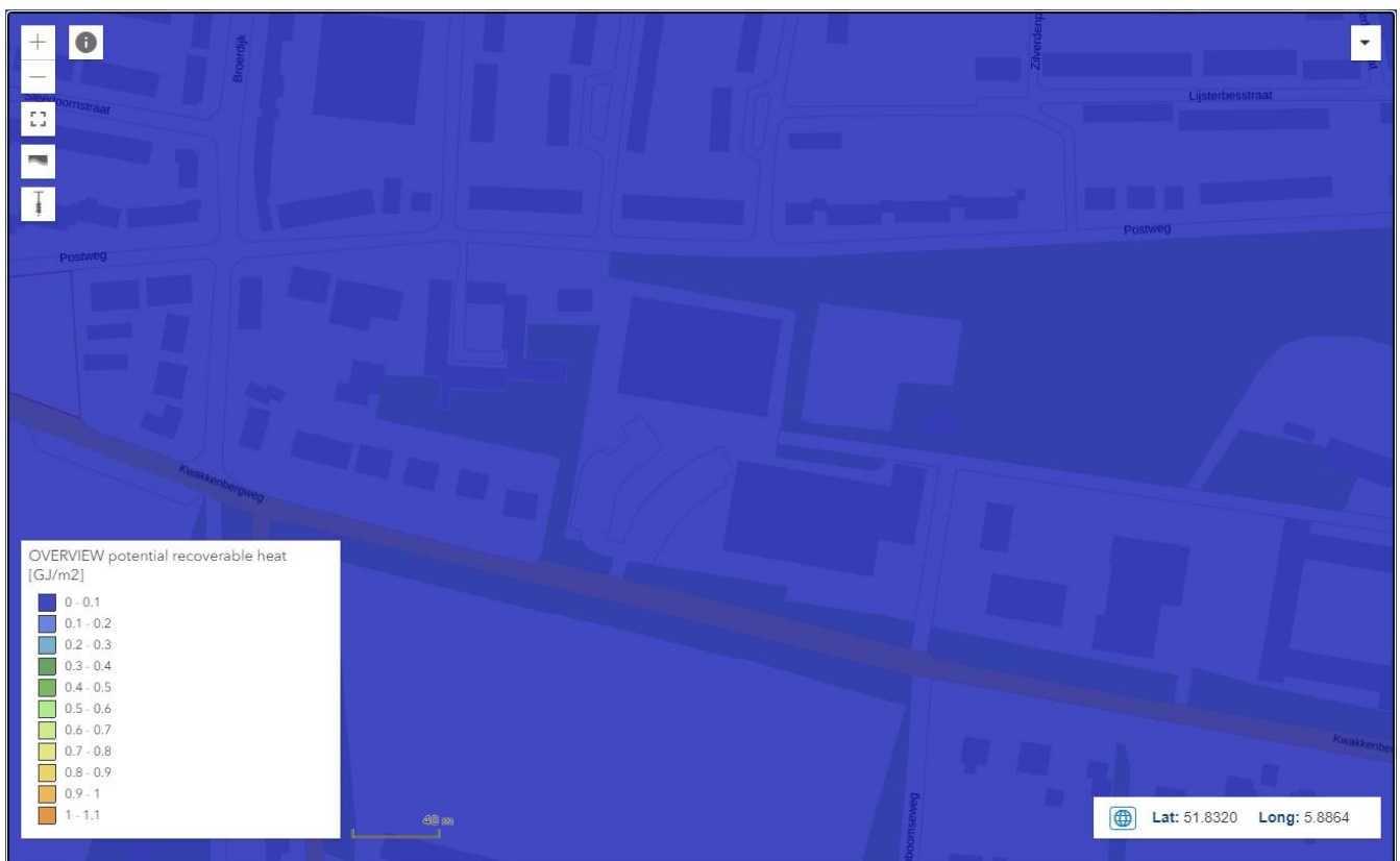
Afbeelding 3, Warmtepotentie Erica Terpstra Sportfondsenbad (Bron: ThermoGIS)
