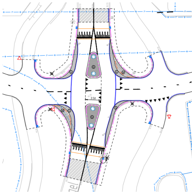
Figuur 1. Ontwerp herinrichting kruispunt
