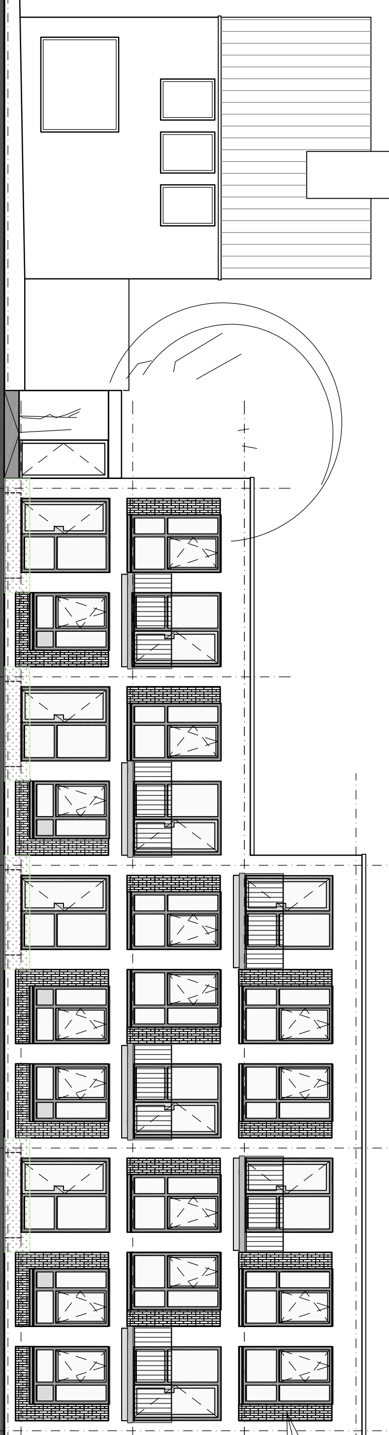
Voorgevel nieuwe toestand GEVEL CERESSTRAAT - OOST
