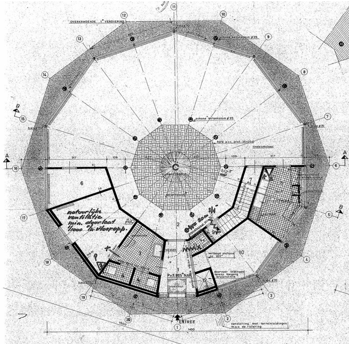
Figuur 3: Definitieve plattegrond begane grond (Regionaal Archief Nijmegen, Digitaal Gebouwen Dossier, inventarisnummer D12.473956, definitieve plattegronden, 2 september 1968).
