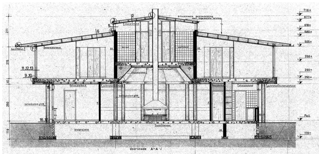
ur 2: Technische doorsnede (Regionaal Archief Nijmegen, Digitaal Gebouwen Dossier, inventarisnummer D12.473942, technische doorsnedes, 2 augustus 1968).
