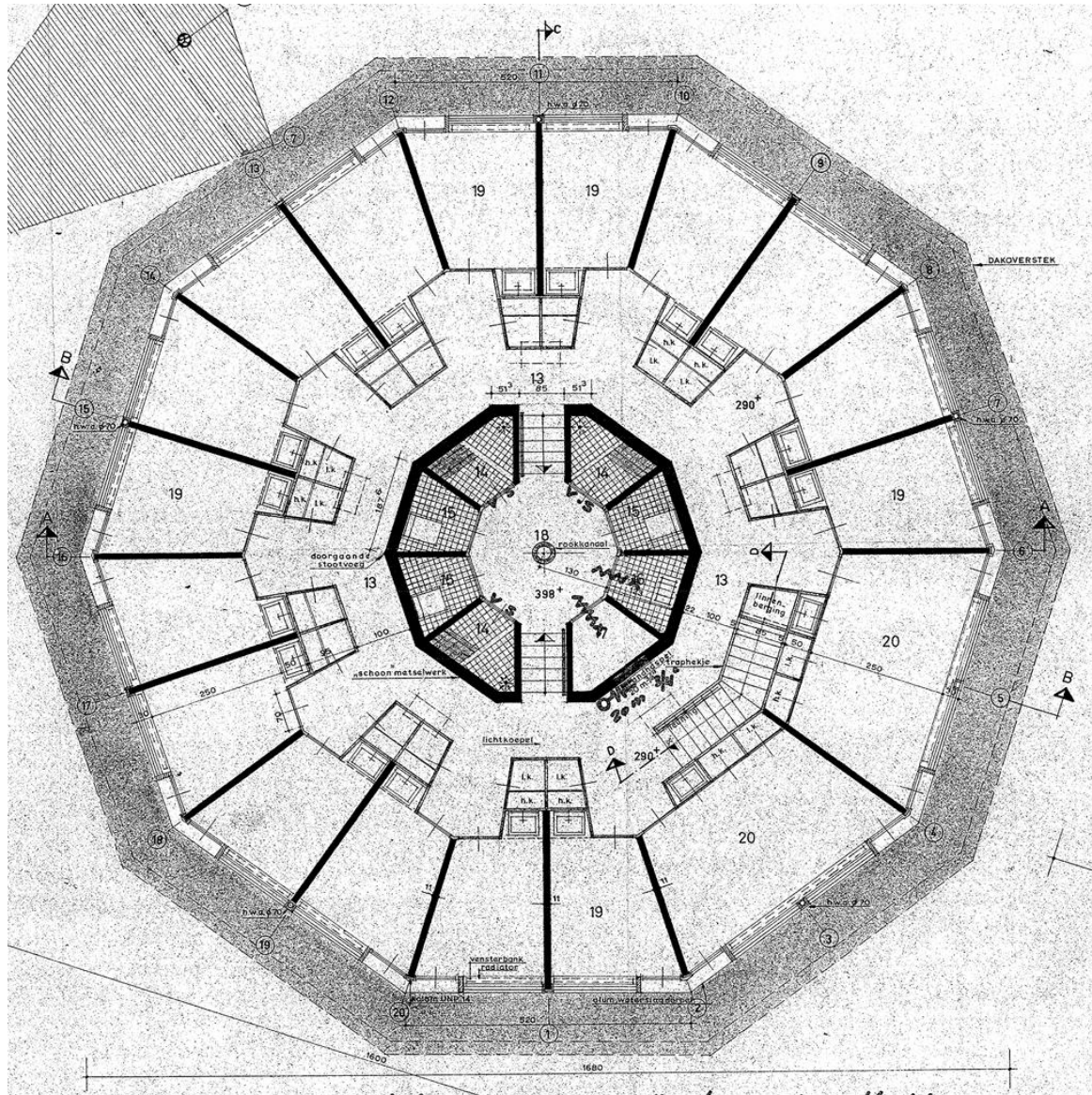
Figuur 4: Definitieve plattegrond verdieping (Regionaal Archief Nijmegen, Digitaal Gebouwen Dossier, inventarisnummer D12.473956, definitieve plattegronden, 2 september 1968).
