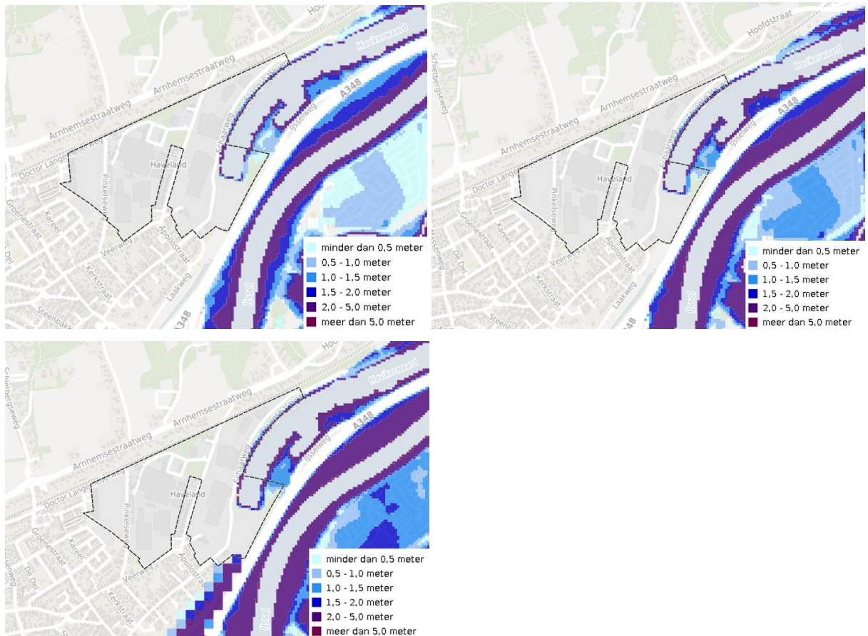
Figuur 3-28 Overstromingsdiepte bij een grote (linksboven); middelgrote (rechtsboven); en kleine (linksonder) kans (bron: Landelijk informatiesysteem water en overstromingen, 2022)
