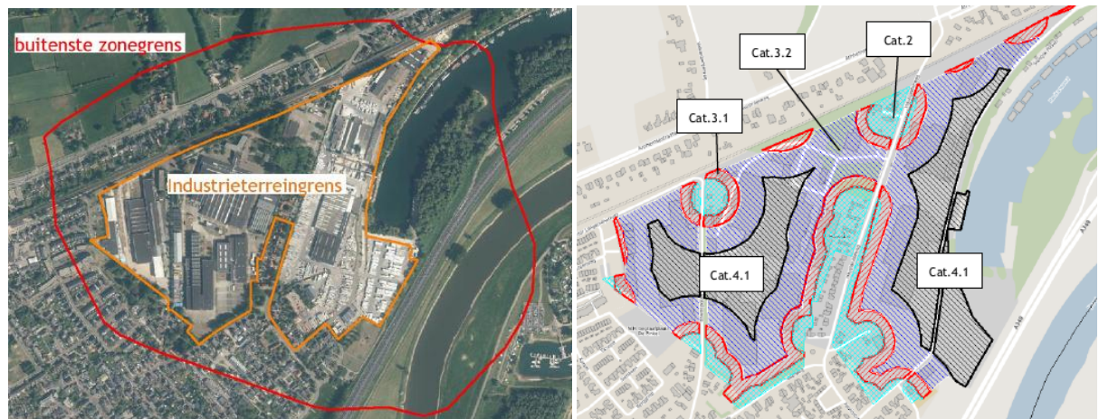
Figuur 3-6 Links: gezoneerde industrieterrein Haveland. Rechts: Milieucategorieën voor milieu-aspecten (anders dan geluid) op industrieterrein volgens bestemmingsplan (bron: DGMR, 2024)
