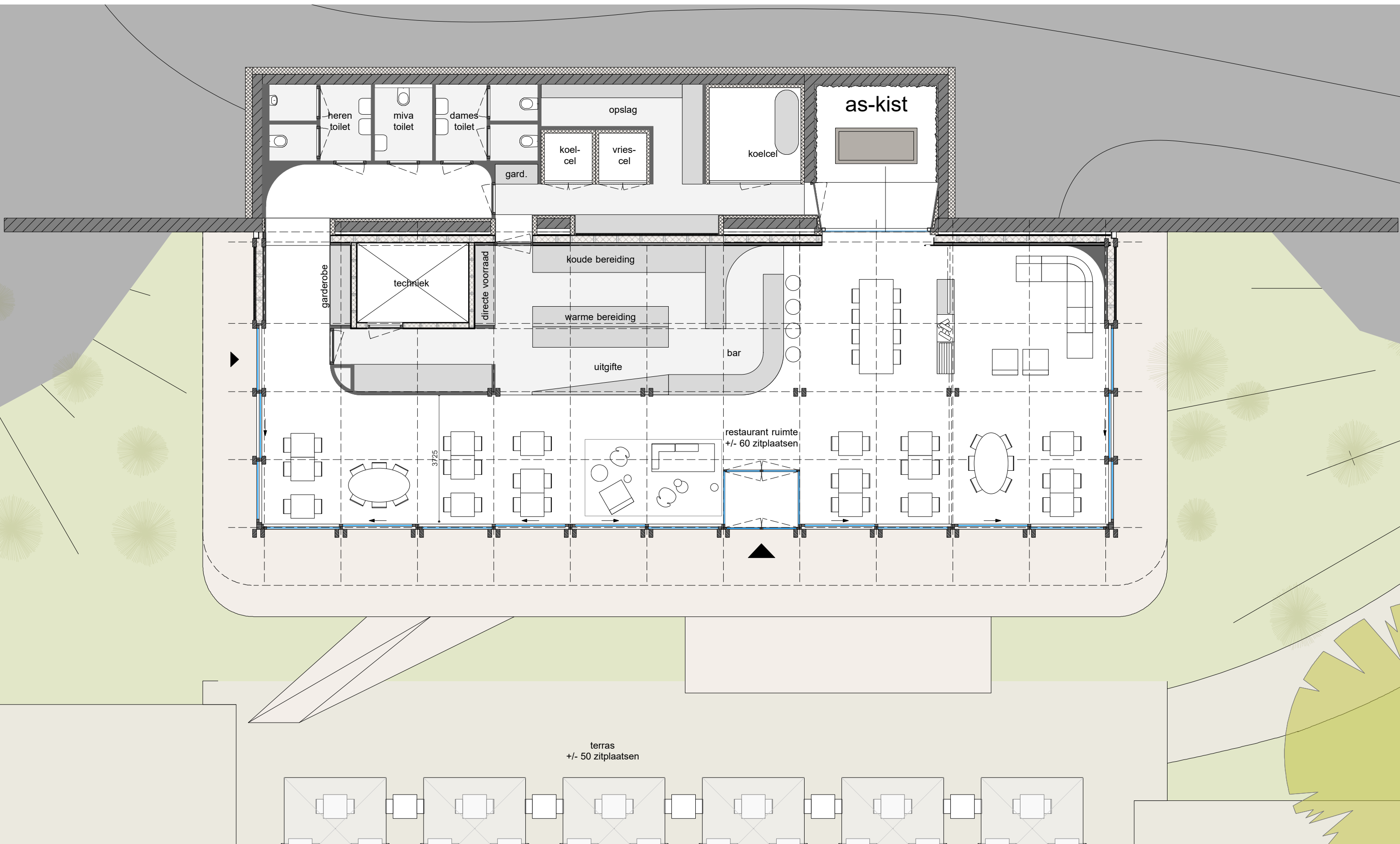
plattegrond | 1:100
