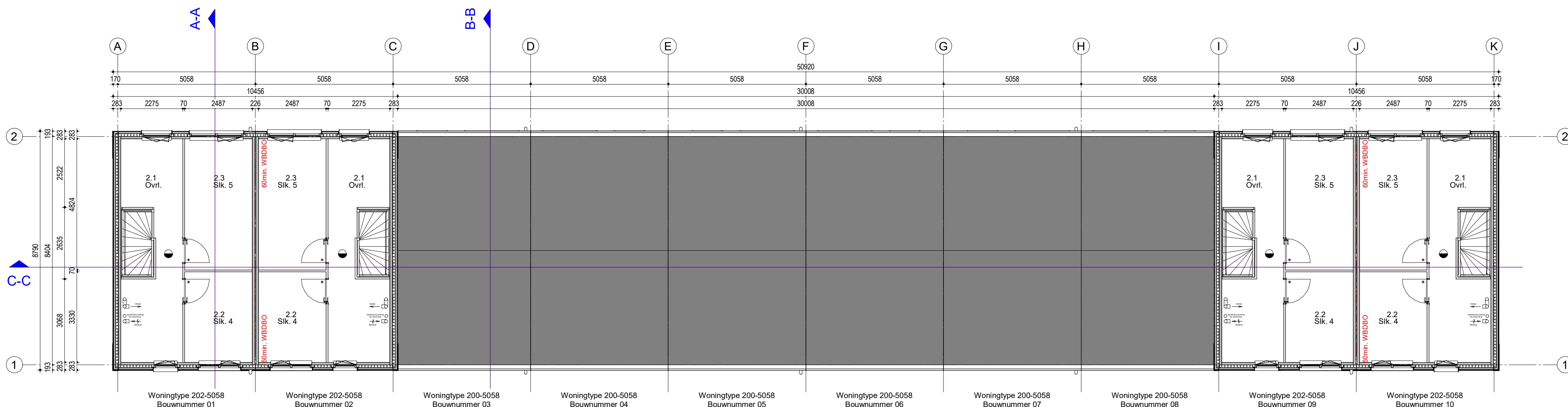
2e Verdieping
