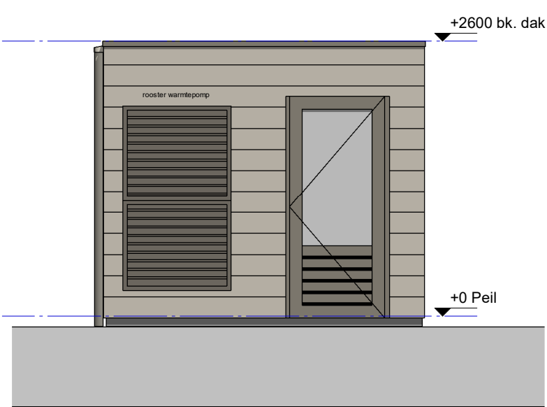
Zijgevel links
