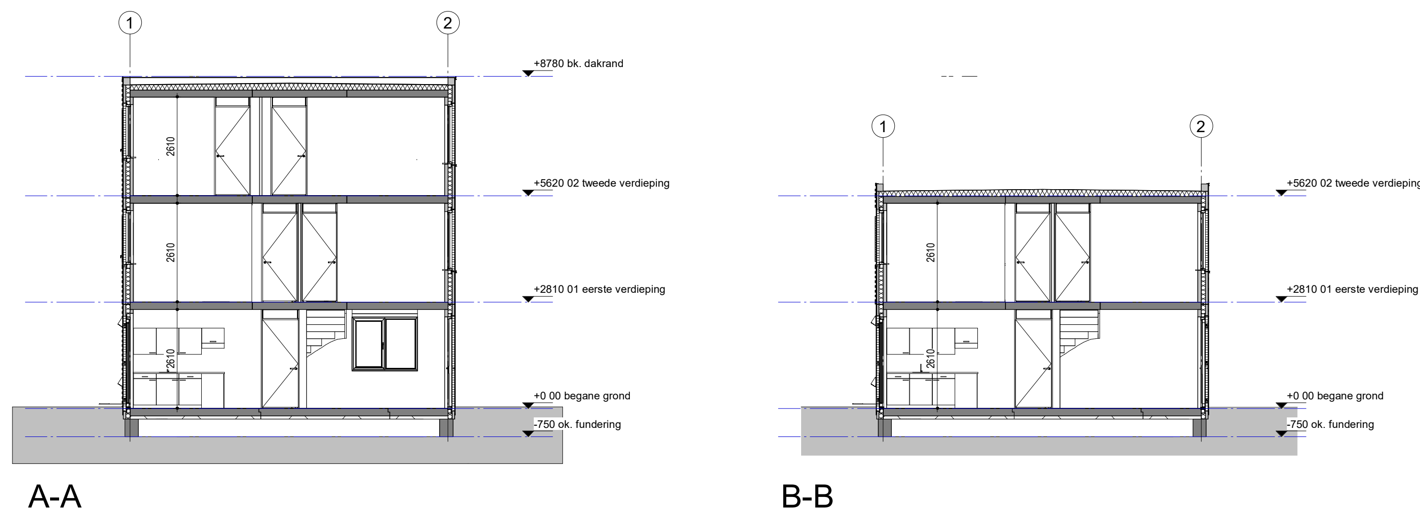
A-A
