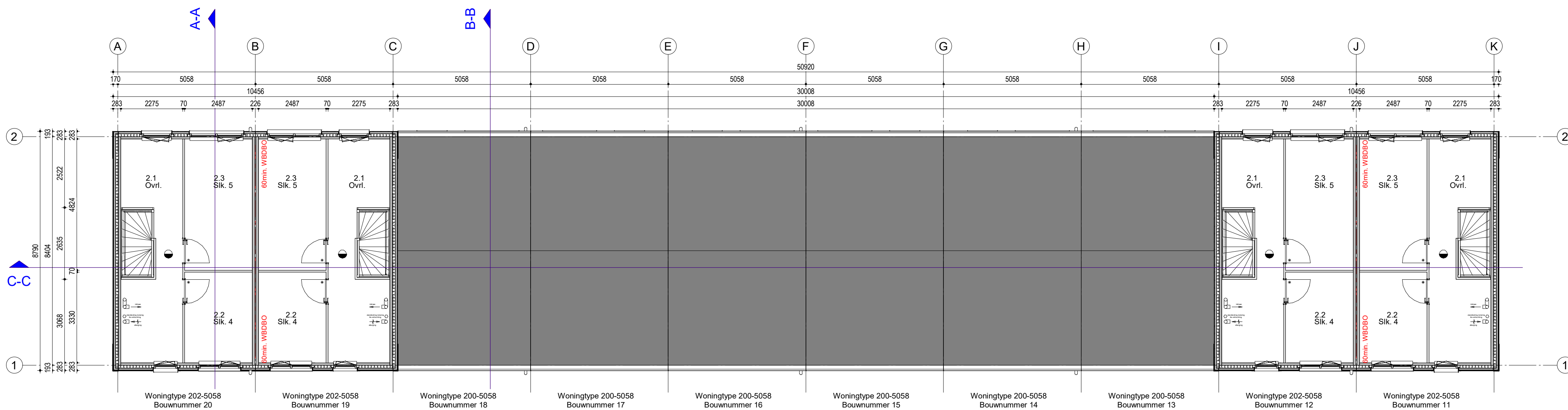
2e Verdieping
