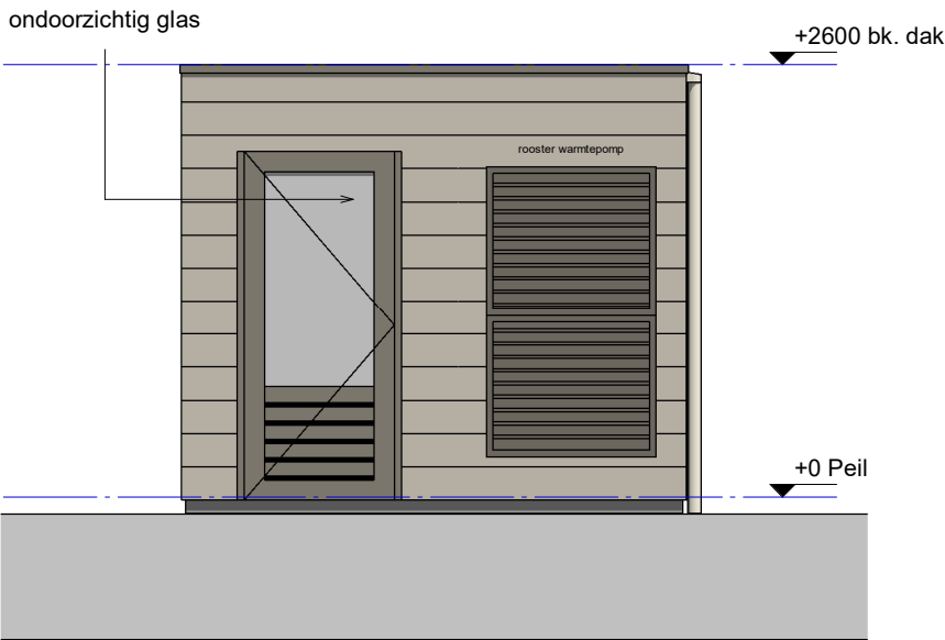
Zijgevel rechts
