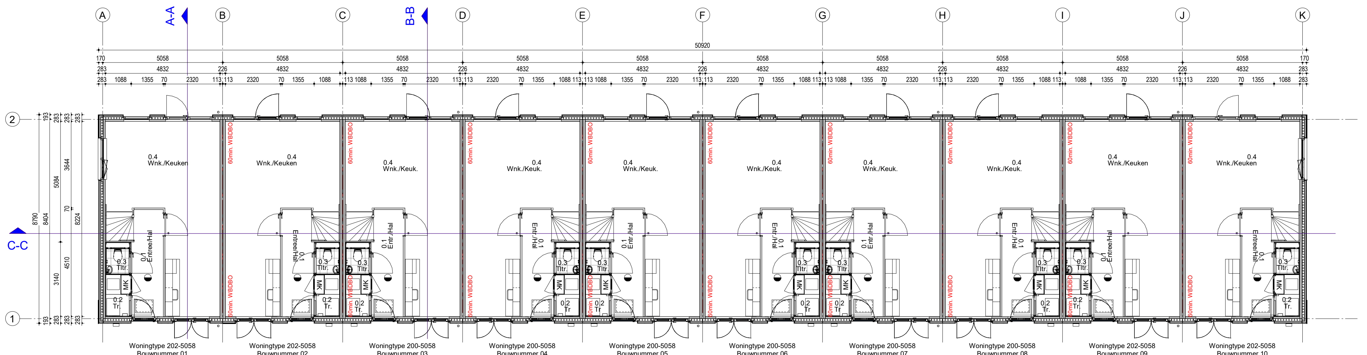
Begane grond
