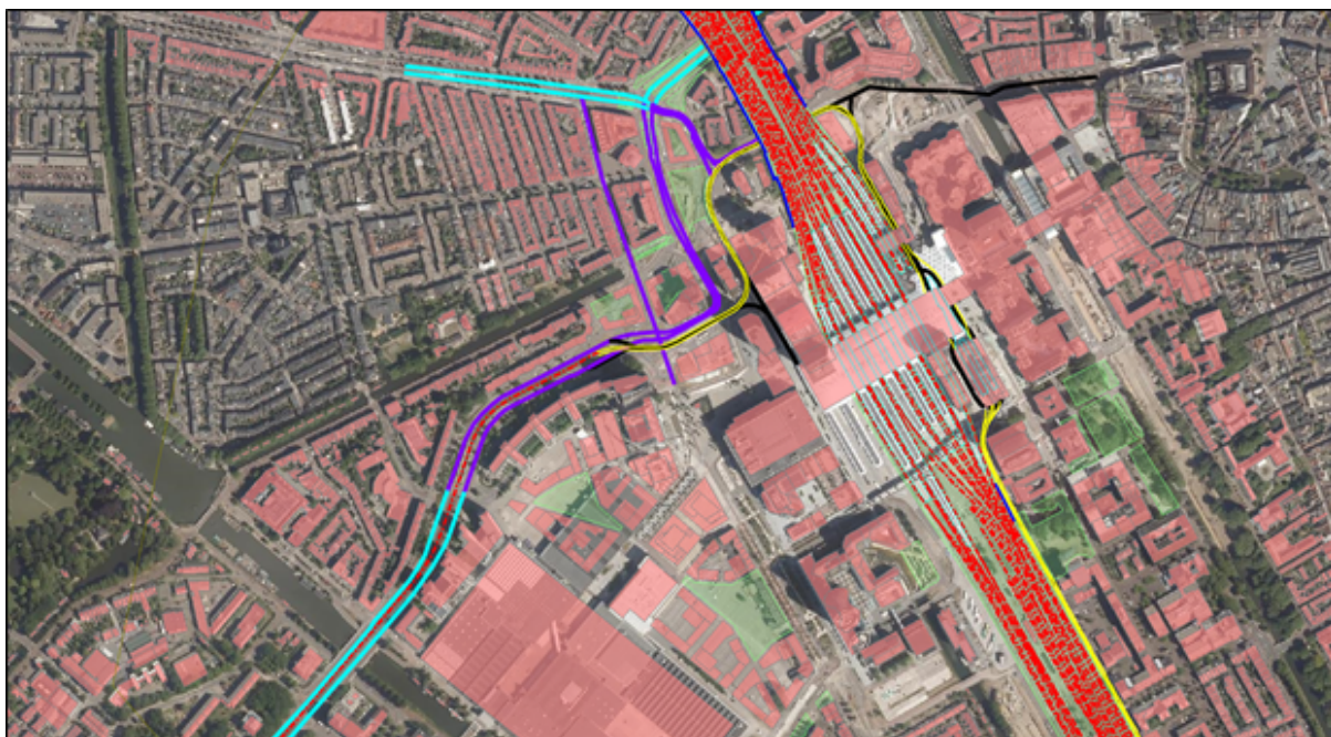
Iding 20: Overzicht rekenmodel weg- en railverkeerslawaai 2D
