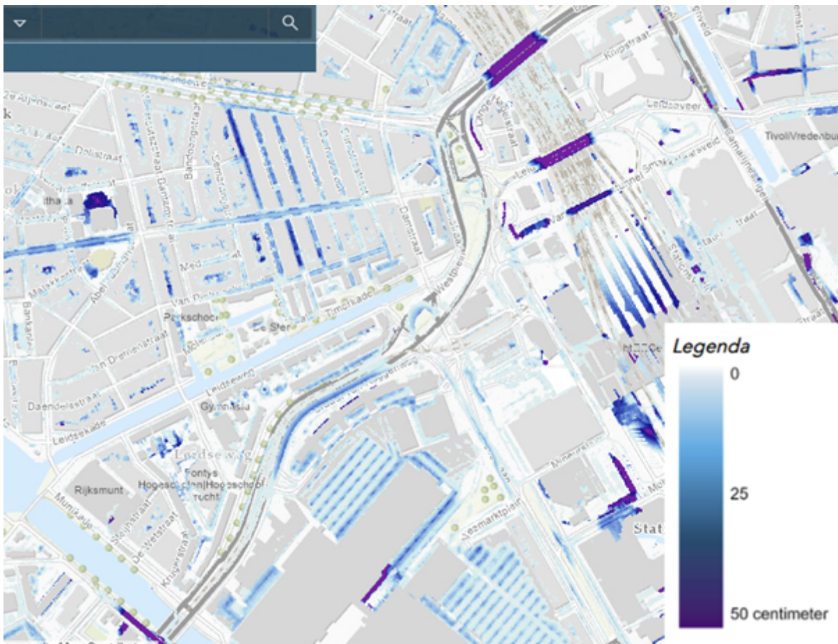
Afbeelding 32: Rekenresultaten water-over-straat berekening bij 80mm blokbui
