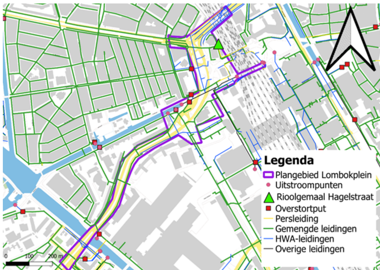
Afbeelding 29: Overzicht bestaande riolering
