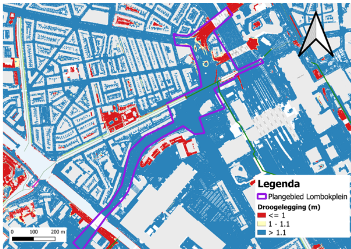
Afbeelding 26: Berekende drooglegging binnen het plangebied
