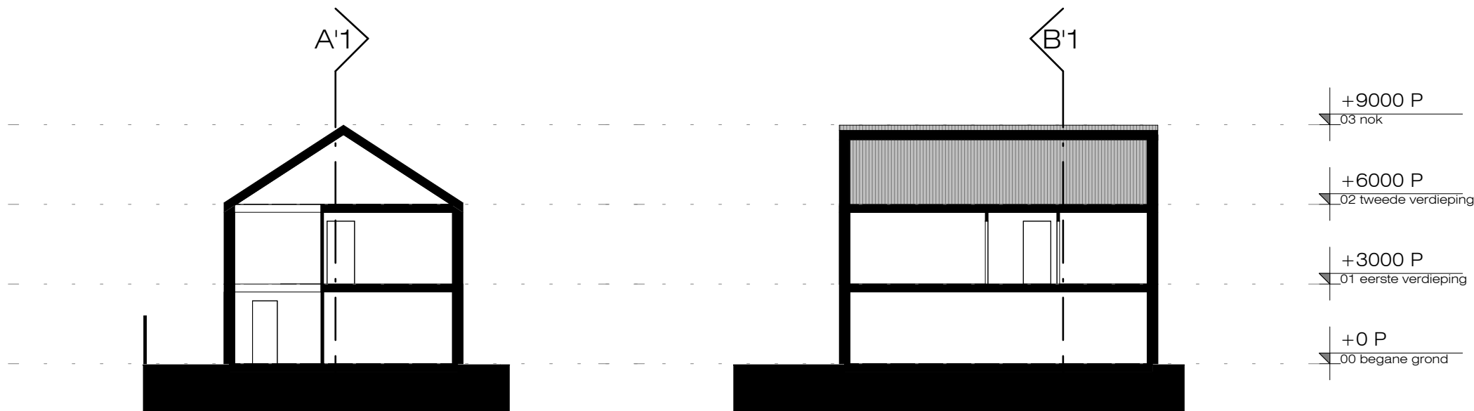
doorsnede B-B
