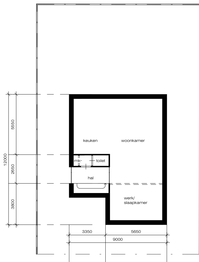
begane grond
