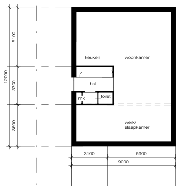
begane grond
