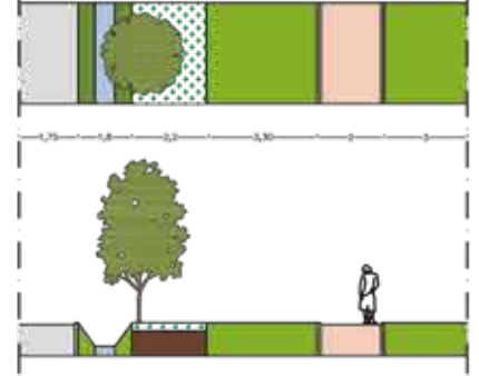
Dwarsprofiel E-E Schaal: 1:250
