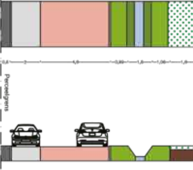
Dwarsprofiel D-D Schaal: 1:250
