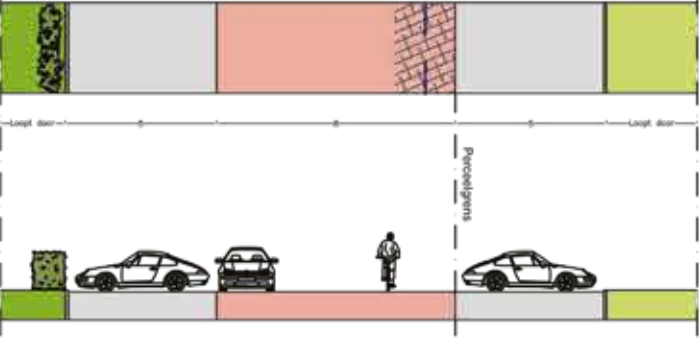
Dwarsprofiel B-B Schaal: 1:250
