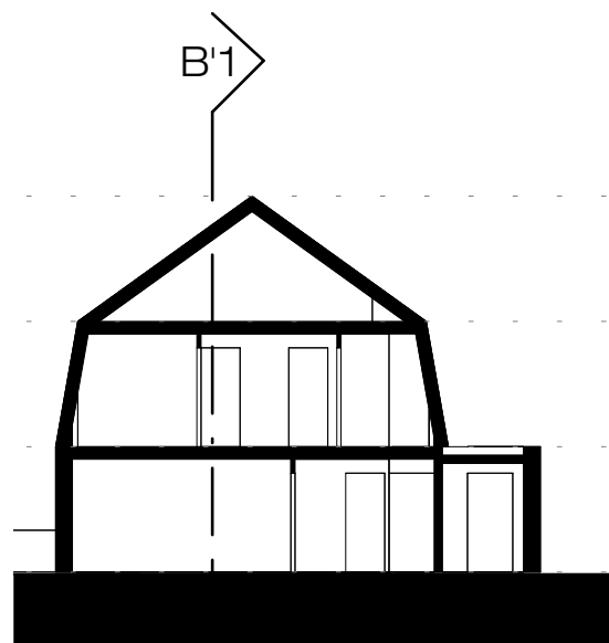
doorsnede A-A
