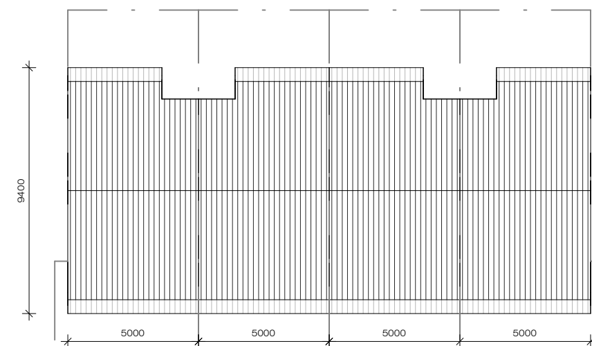
dakverdieping
