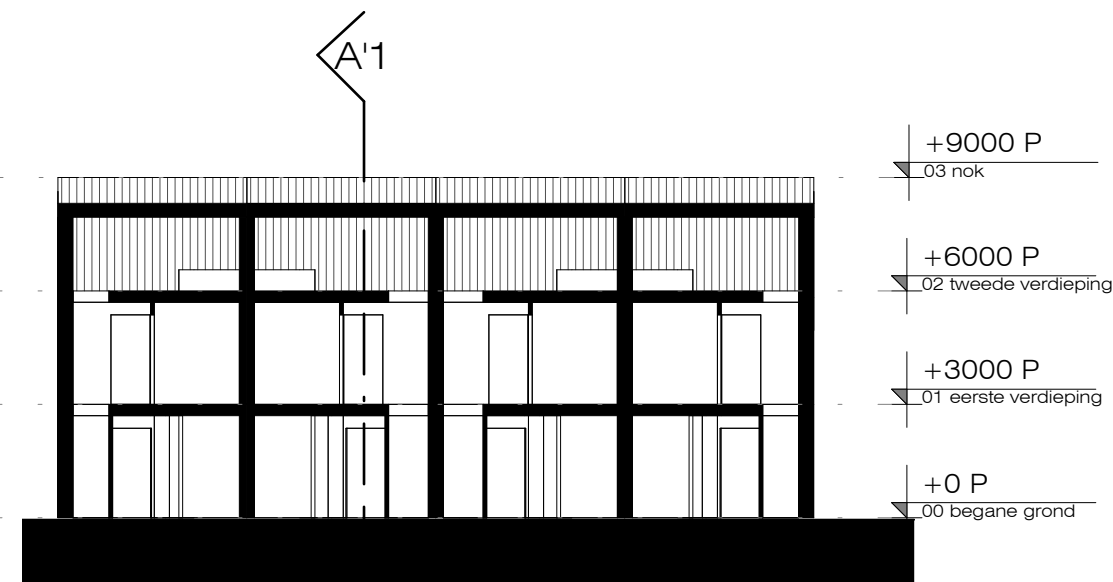
doorsnede B-B
