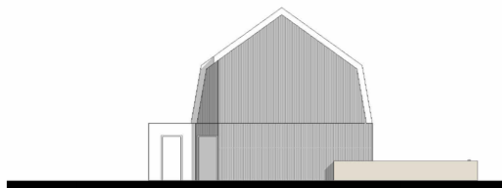
rechter zijgevel
