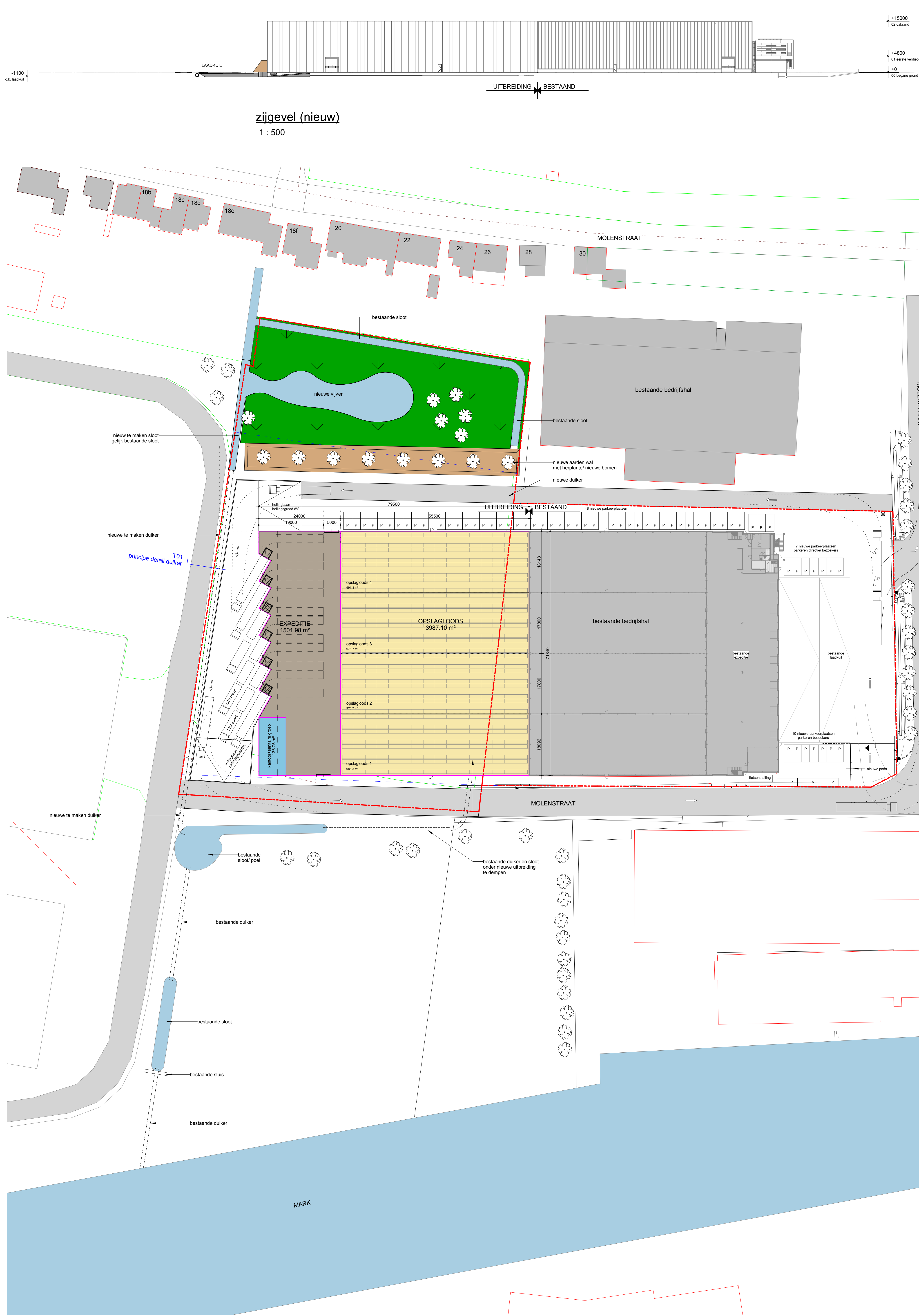
plekkenplan uitbreiding 1 : 500
