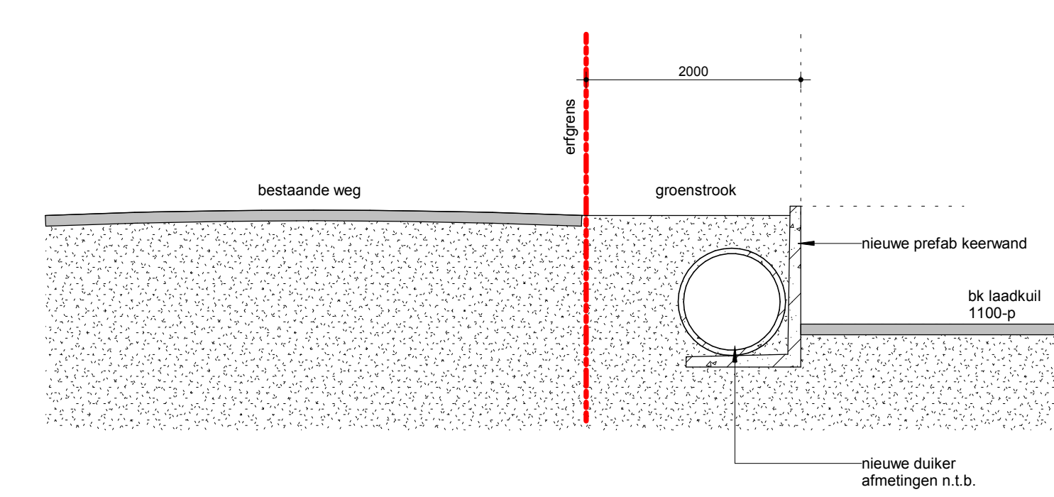
T01 principe detail duiker 1 : 50
