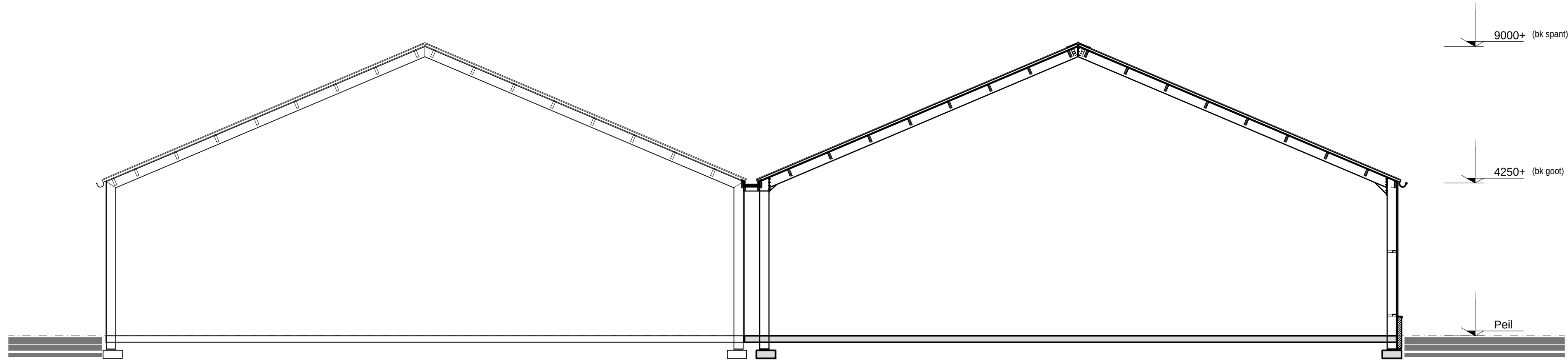
doorsnede A-A
