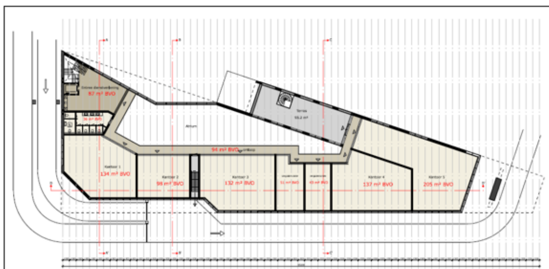
Afbeelding 3.9: plattegrond verdieping (bron: EVE architecten)
