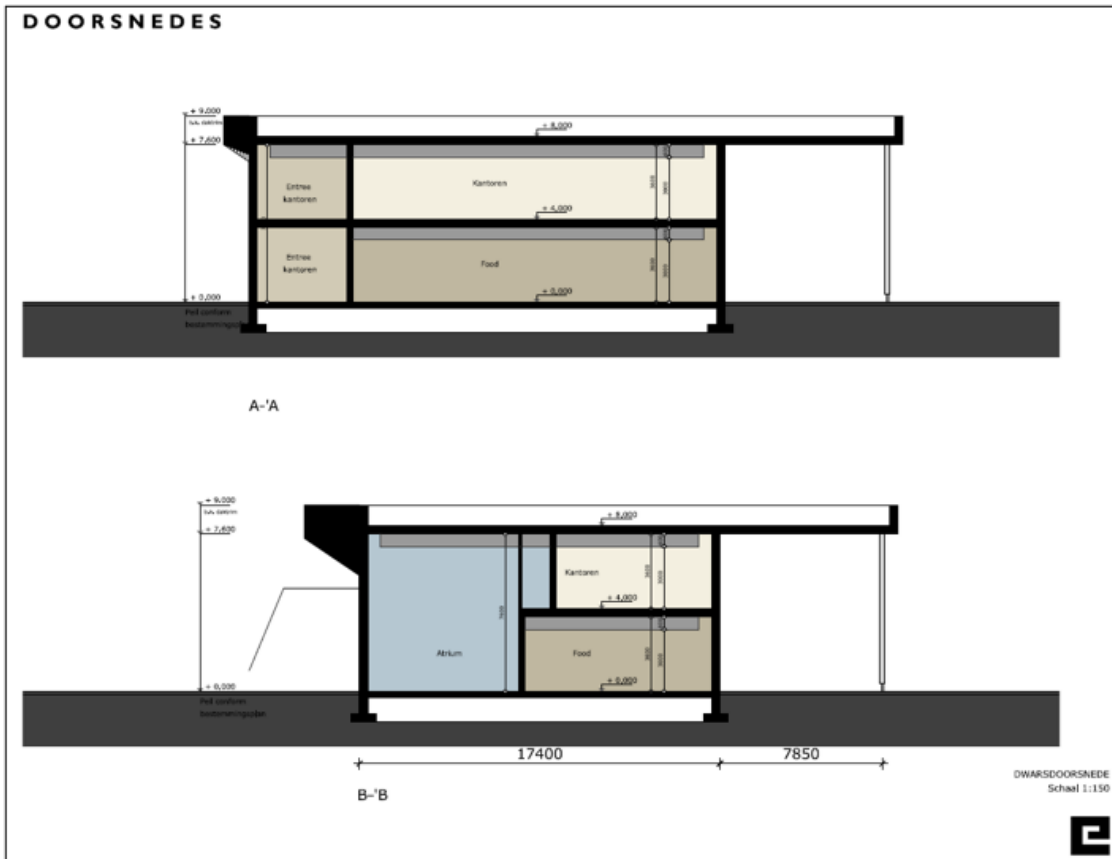
Afbeelding 3.7: dwarsdoorsnedes van het gebouwwontwerp met hoogten (bron: EVE architecten)
