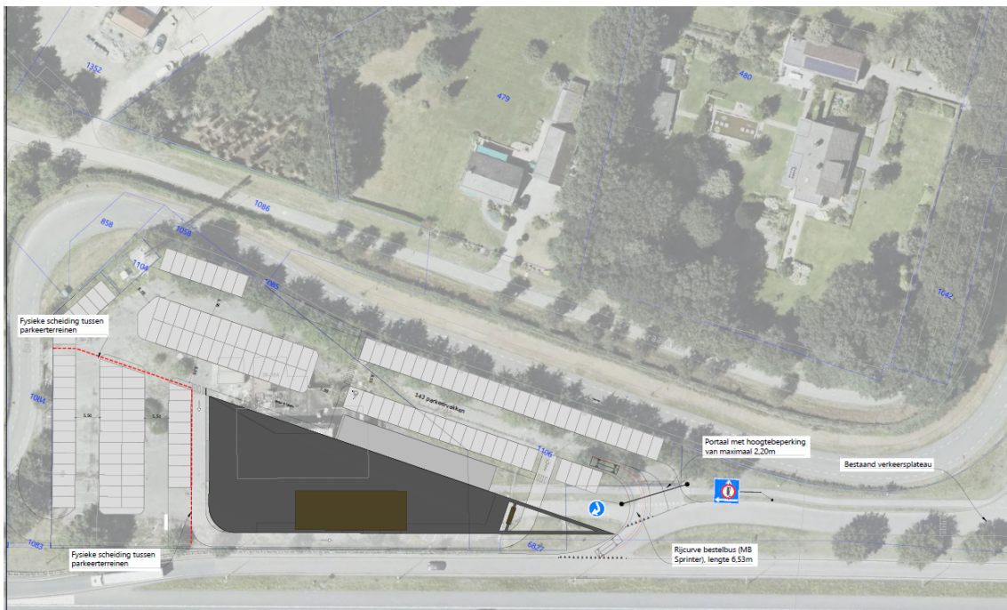
Afbeelding 3:10 schetsvoorstel terreininrichting interne infrastructuur + parkeervoorzieningen (bron: Goudappel Coffeng)
