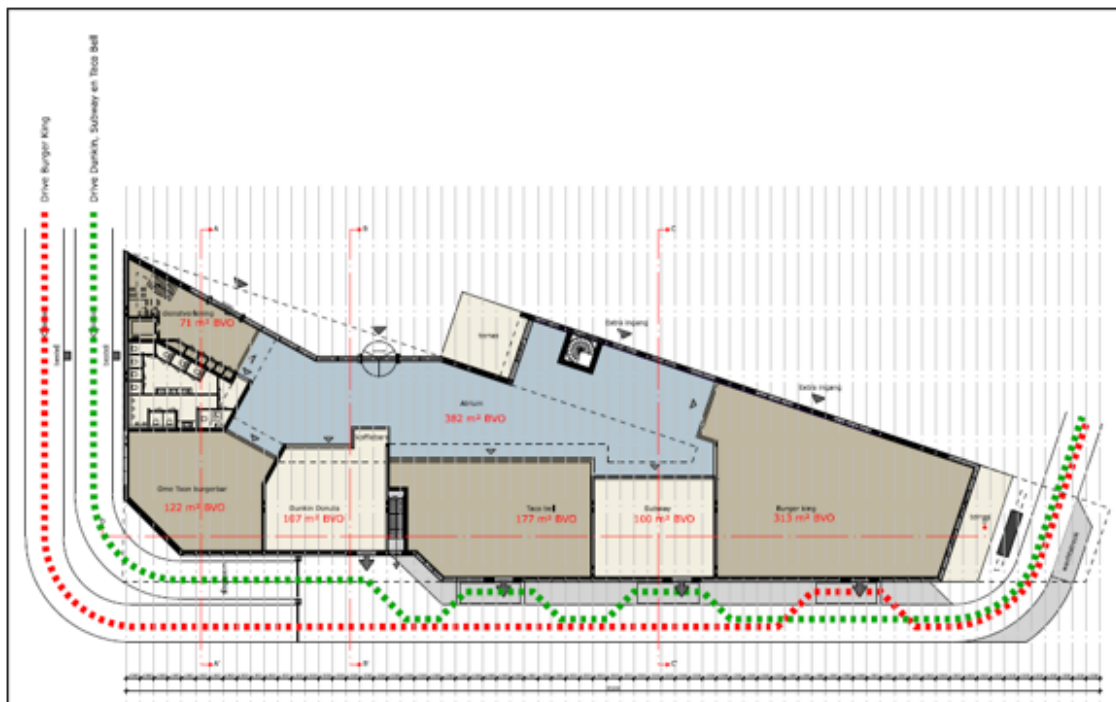
Afbeelding 3.8: plattegrond indeling begane grondlaag (bron: EVE architecten)
