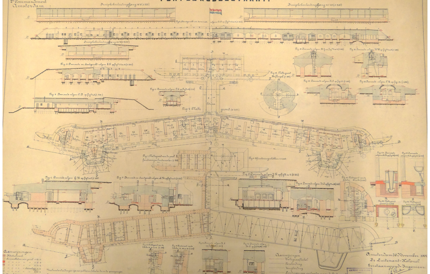
PLATTEGRONDTEKENING MET DOORSNEDEN EN DETAILS UIT 1905 VAN HET FORT. (ARCHIEF WWW.STELLING-AMSTERDAM.NL/R.ROS)
