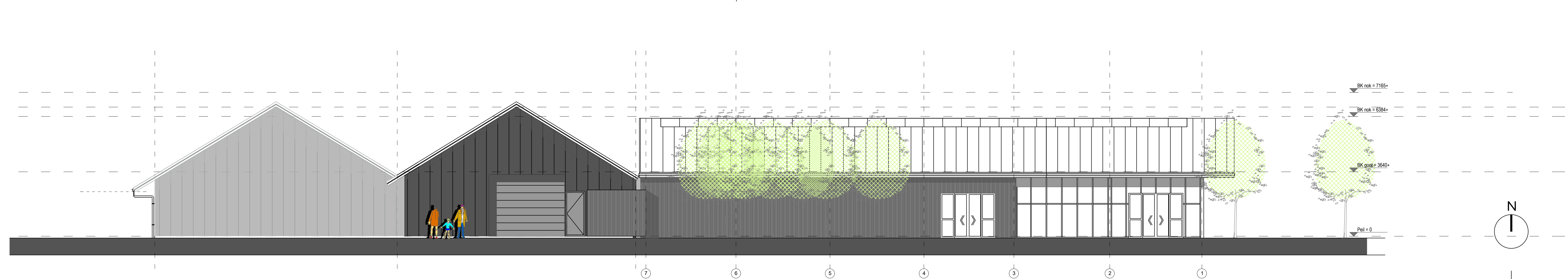
Ontwerp zuidgevel (voorgevel)
