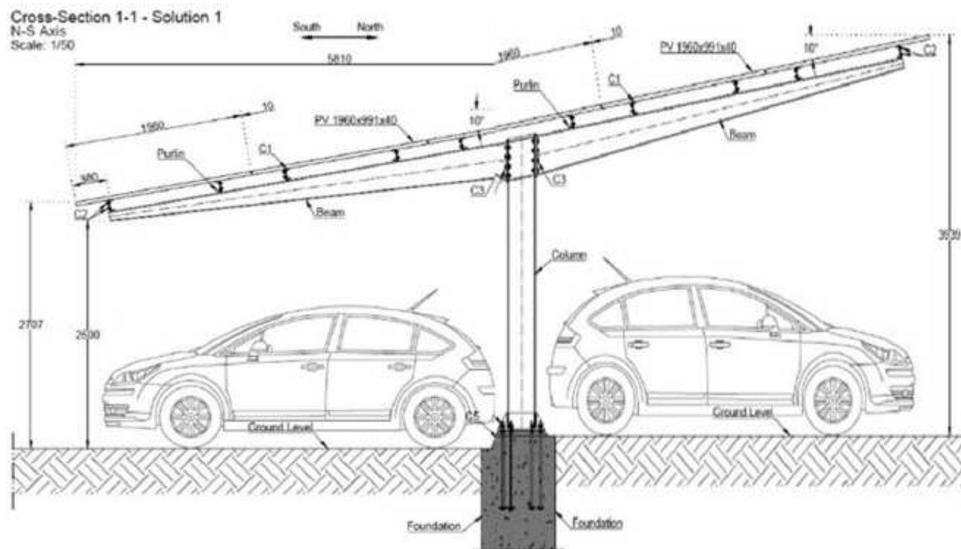
Figuur 13: Een constructietekening van de voorziene carport.
