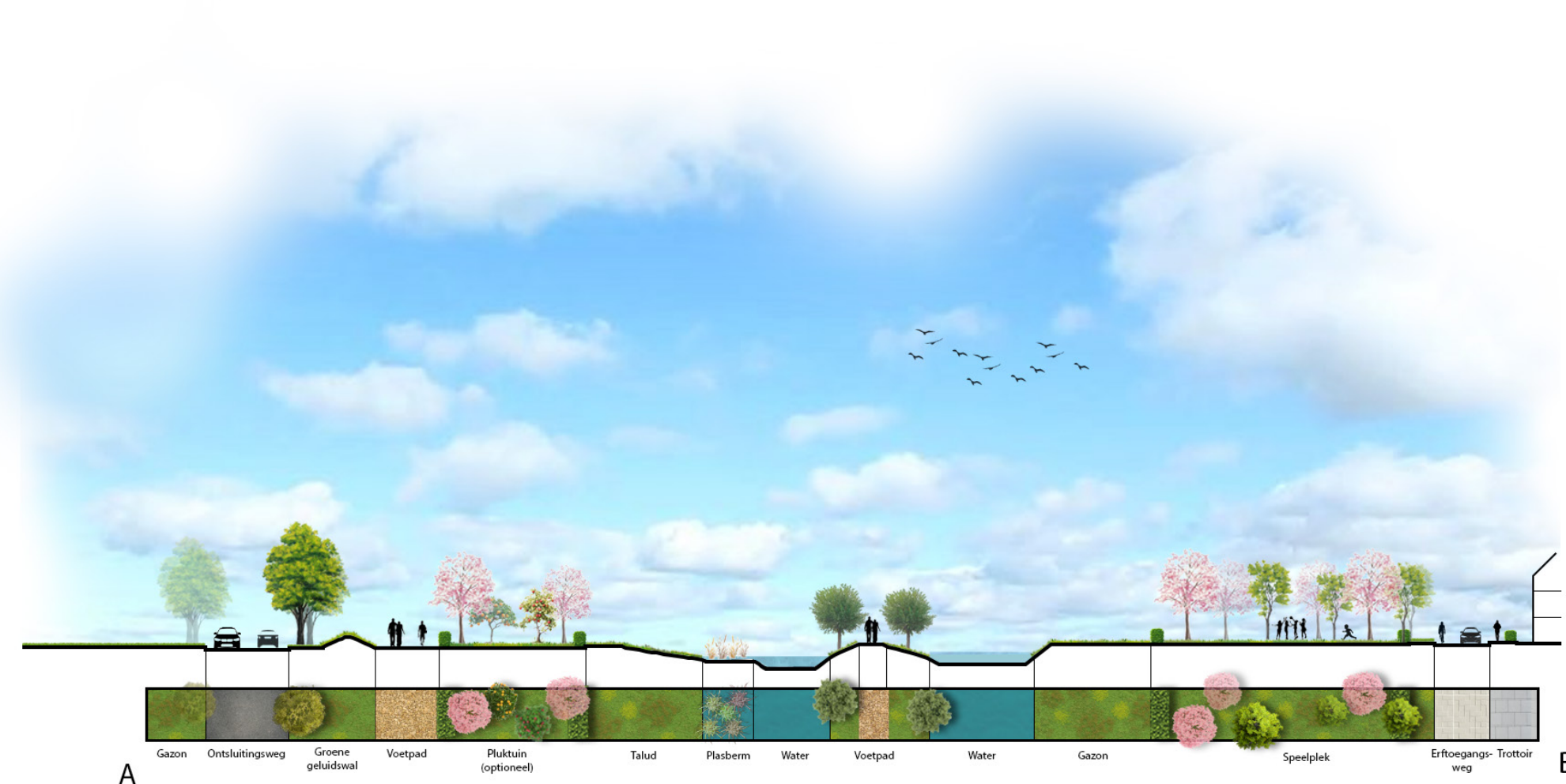
Profielen met de belangrijkste elementen
