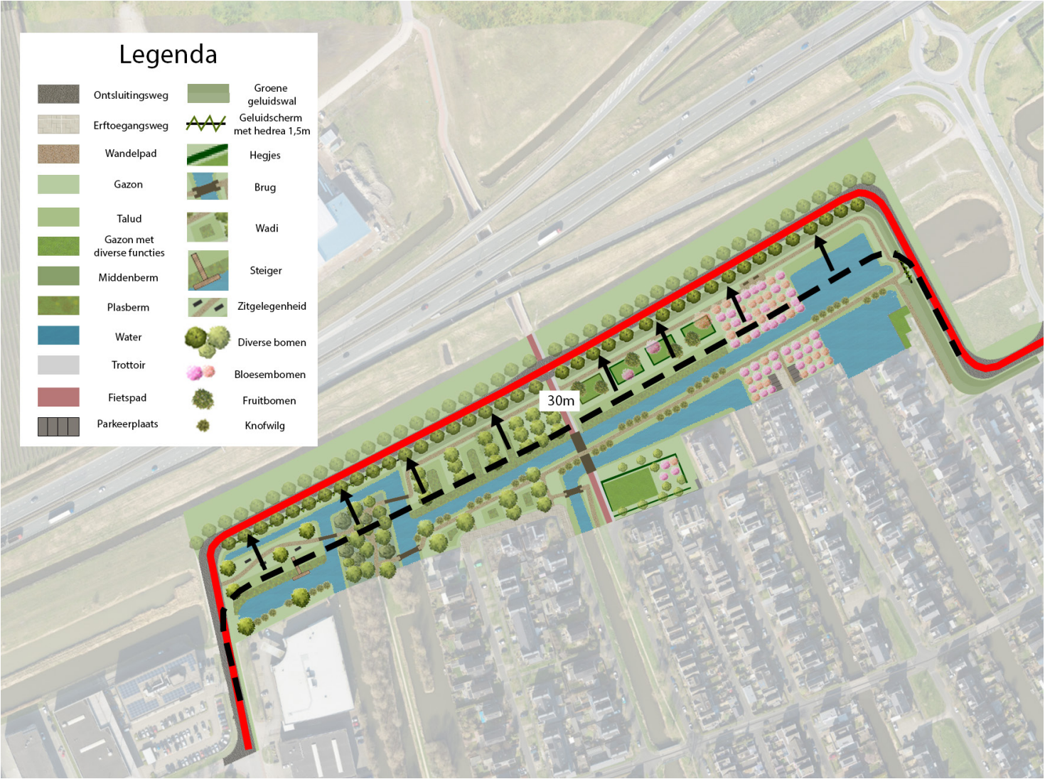
Verleggen van de rijbaan
