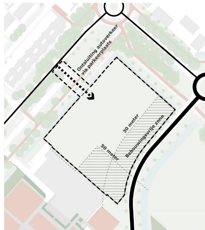
Figuur 27: richtafstanden naastgelegen tennisvereniging en toegang autoverkeer naar plangebied
