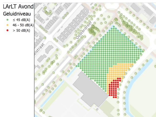
Figuur 28: Beeld uit het concept geluidsonderzoek. Geluidsniveau in de avondperiode (zonder maatregelen).
