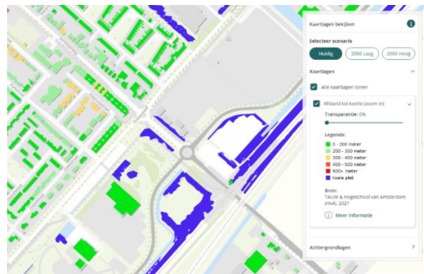
Figuur 26: Screenshot uit de kaartviewer van de klimateffectatlas. De zwembadlocatie vervult de functie van een koelteplek.
