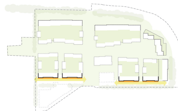
Stadsstraat met verspringende rooilijn en een Delftse stoep
