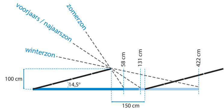
Schaduwwerking bij een zuid-opstelling van 1 meter hoog.
