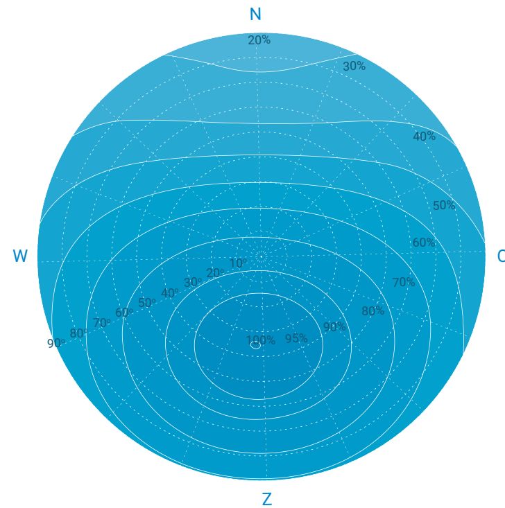
Zonne-instralingsdiagram voor Nederland wat de relatie tussen oriëntatie, hoek van het paneel en efficiëntie van het paneel laat zien.
