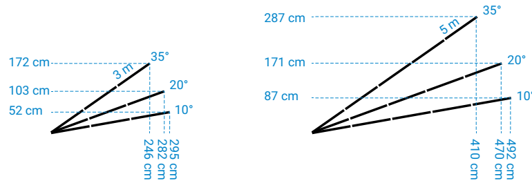
Hoogte en ruimtebeslag bij opstellingen onder diverse hoeken voor 3 liggende panelen (links) en 5 liggende panelen (rechts)
