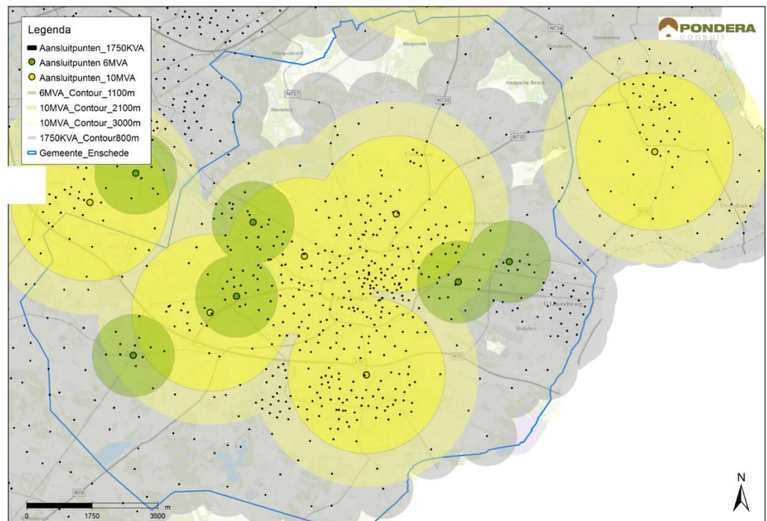
Figuur 4.3 Aansluitmogelijkheden op het elektriciteitsnetwerk en afstandscontouren zonnevelden
