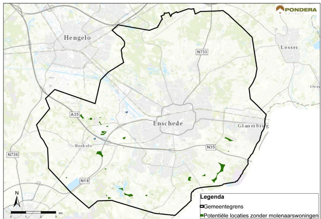
Figuur 4.5 Theoretisch mogelijke locaties voor windturbines (circa 150 meter tiphoogte) in Enschede o.b.v. harde belemmeringen
