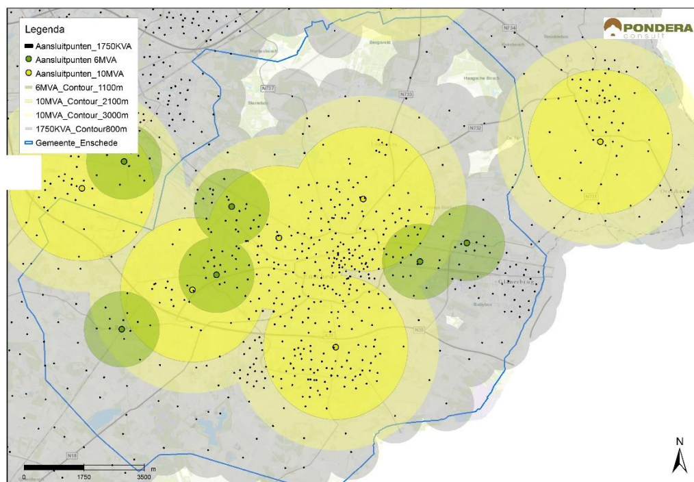
Figuur 12.2 Afstanden tot netaansluitingsmogelijkheden van ENEXIS
