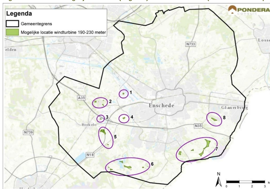
Figuur Theoretisch mogelijke locaties (in groen) voor windturbines (190 – 230 meter tiphoogte)
