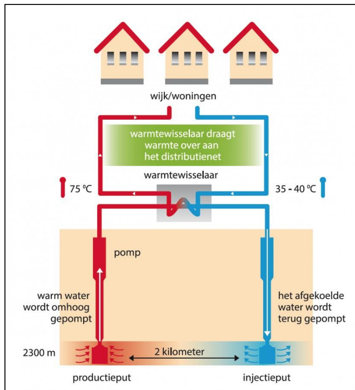
Figuur 4.6 Principe van de inzet van geothermie
