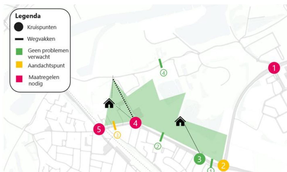
Figuur 0.1: Westervoort Noord en locaties van kruispunten met voorgestelde maatregelen
