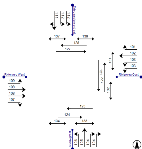
Figuur 4.3: Signaalgroepen kruispunt Rivierweg – Driegaardensestraat
