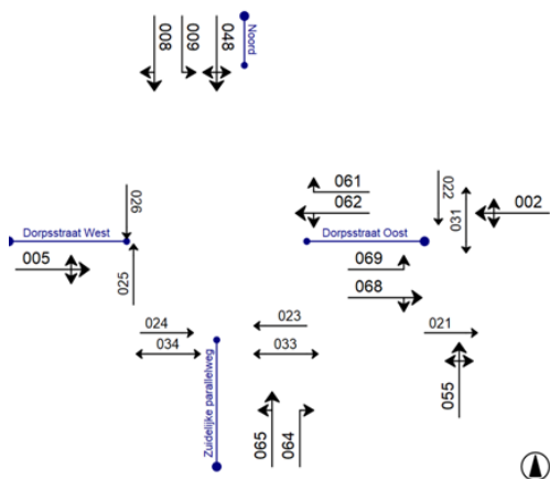
Figuur 4.9: Signaalgroepen kruispunt Brugweg – Dorpstraat
