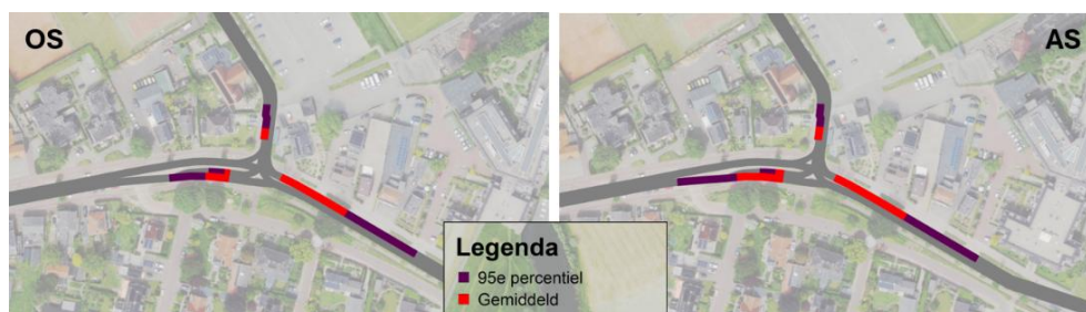
Figuur 4.7: Resultaten VISSIM simulatie met een linksafvak van west naar noord waarop 3 auto's zich op kunnen stellen
