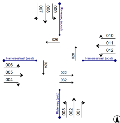
Figuur 4.4: Signaalgroepen kruispunt Hamersestraat - Rivierweg
