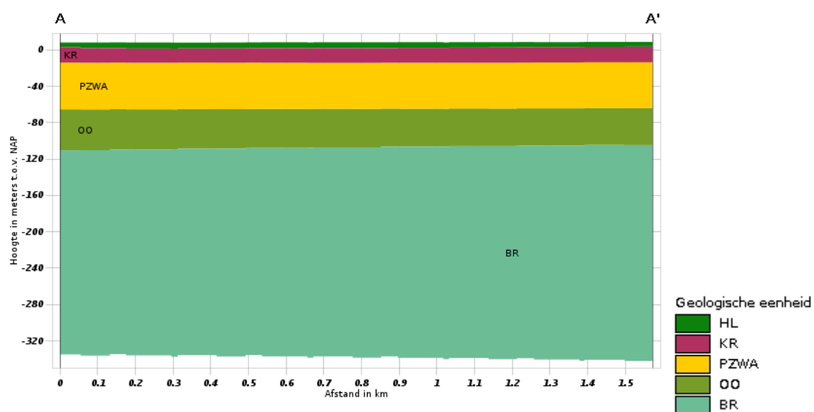
Figuur 3: Landelijk model DGM v2.2 (bron 4c)
