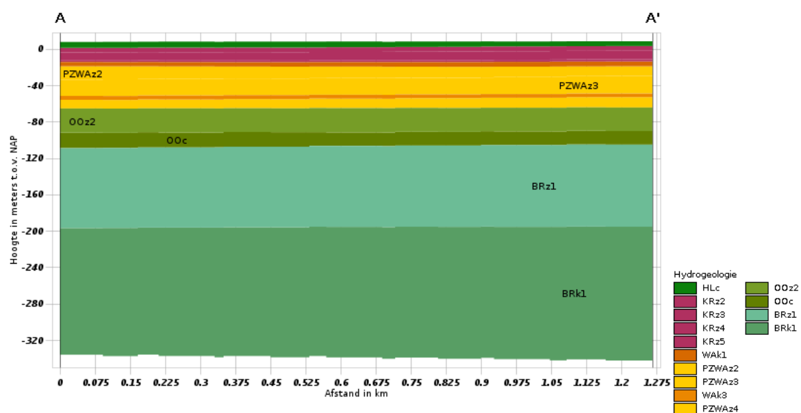
Figuur 2: Geohydrologisch model gebaseerd op REGIS II.1 (bron 4c)
