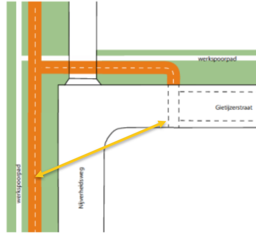
Figuur 4.22 Principe voorrang Nijverheidsweg/Giet- ijzerstraat
