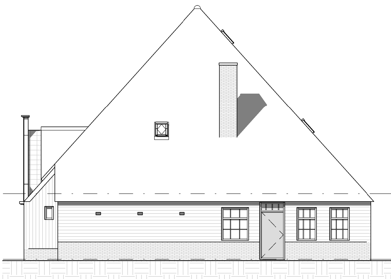
Rechter zijgevel bestaande en nieuwe situatie
