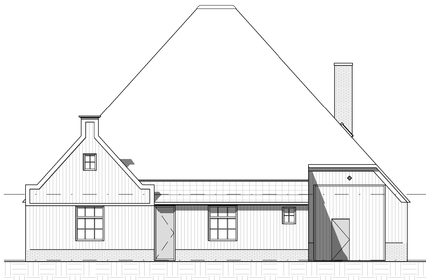
Voorgevel bestaande en nieuwe situatie
