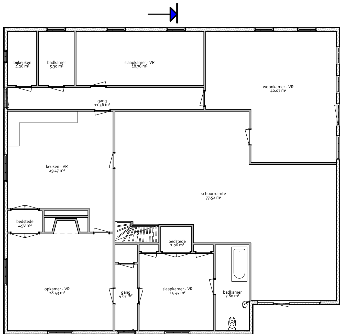
BG bestaande situatie
