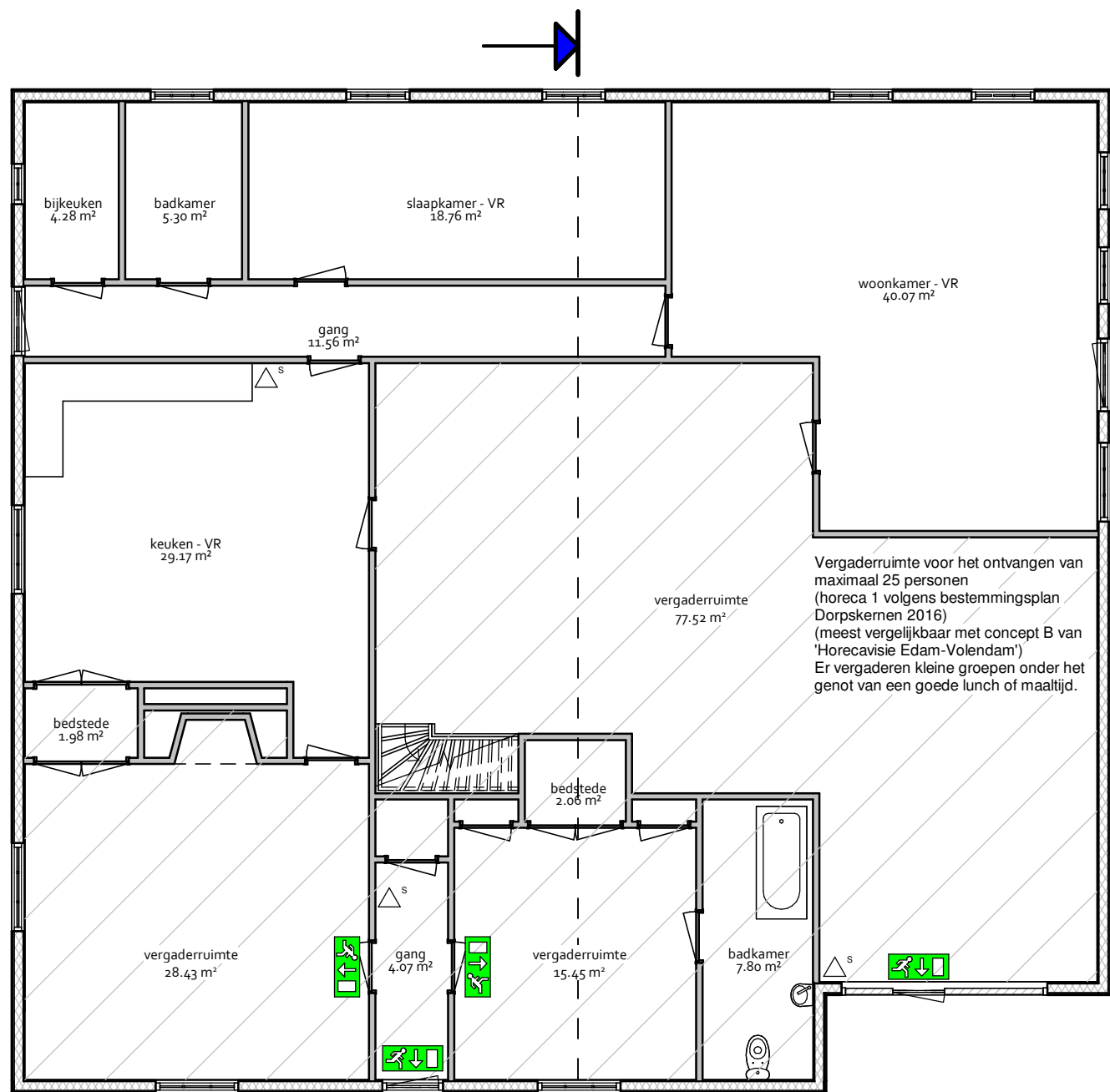
BG nieuwe situatie
