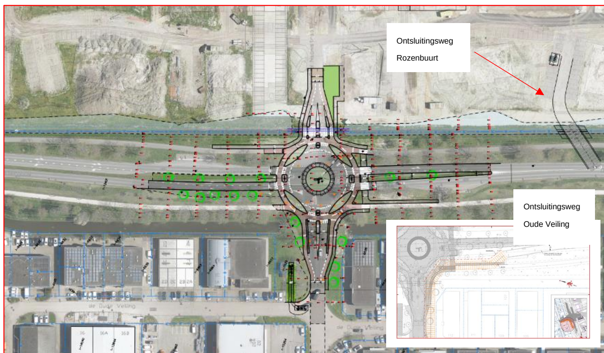
Figuur 1 Ontwerp rotonde en tijdelijke weg Rozenbuurt en Bedrijventerrein
