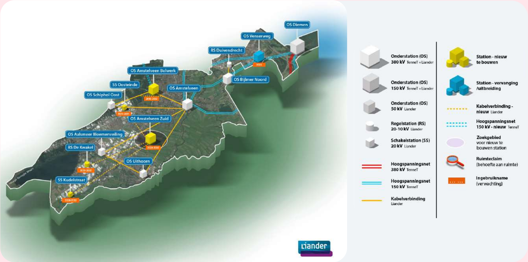
Amstelland Netsituatiekaart van Amstelland (>2MW)
