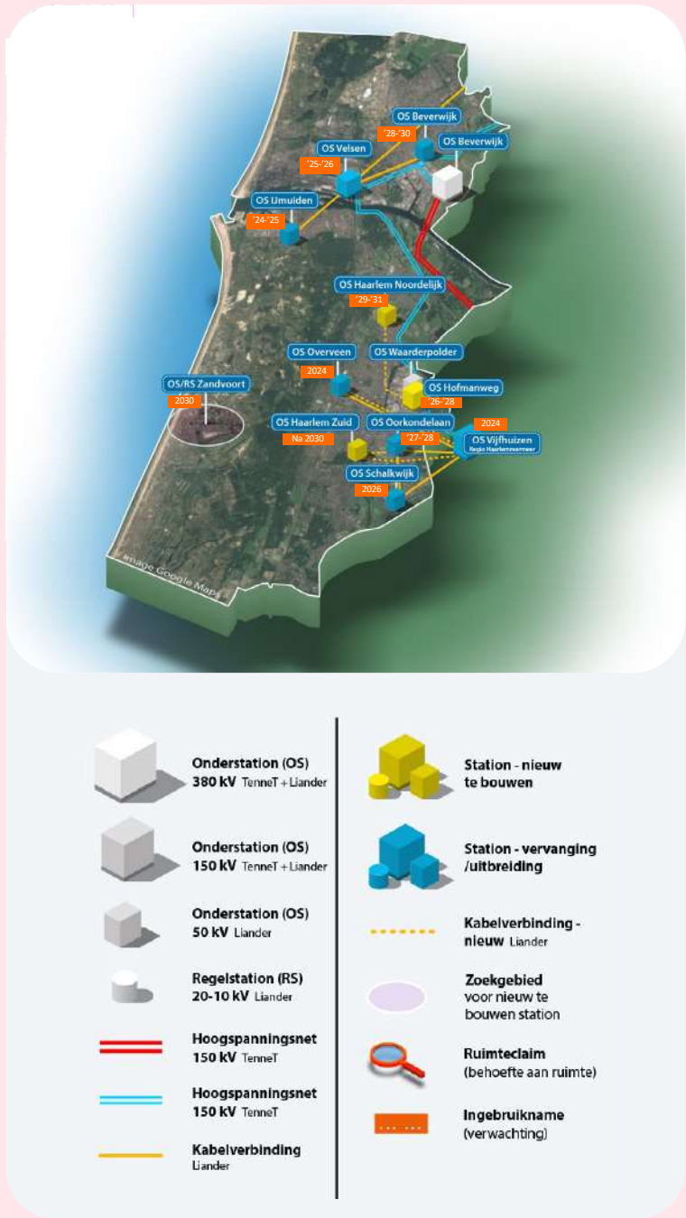
Netsituatie van IJmond & Zuid-Kennemerland (>2MW, huidig en voorzien)
