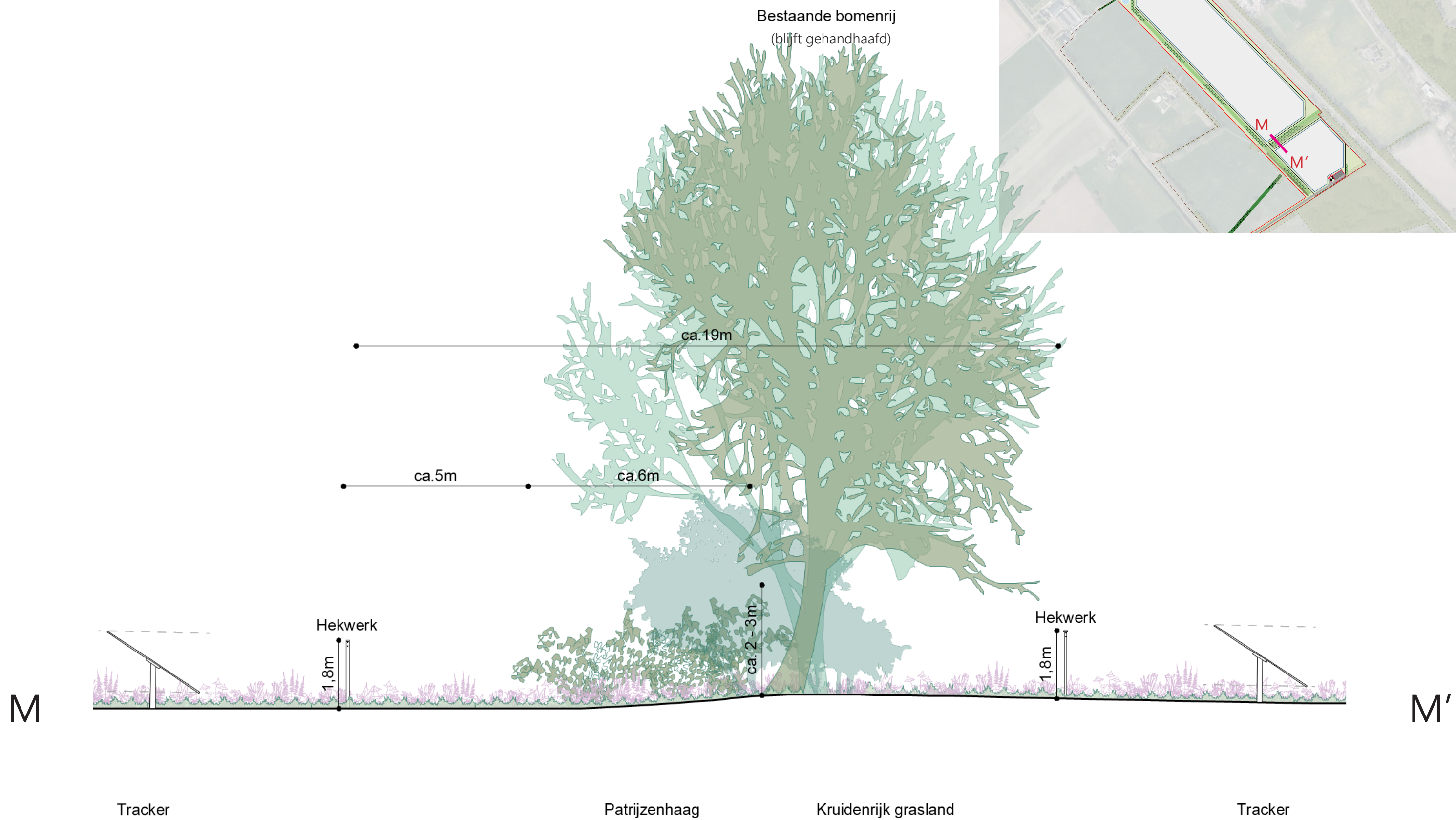
Doorsnede M - M'
