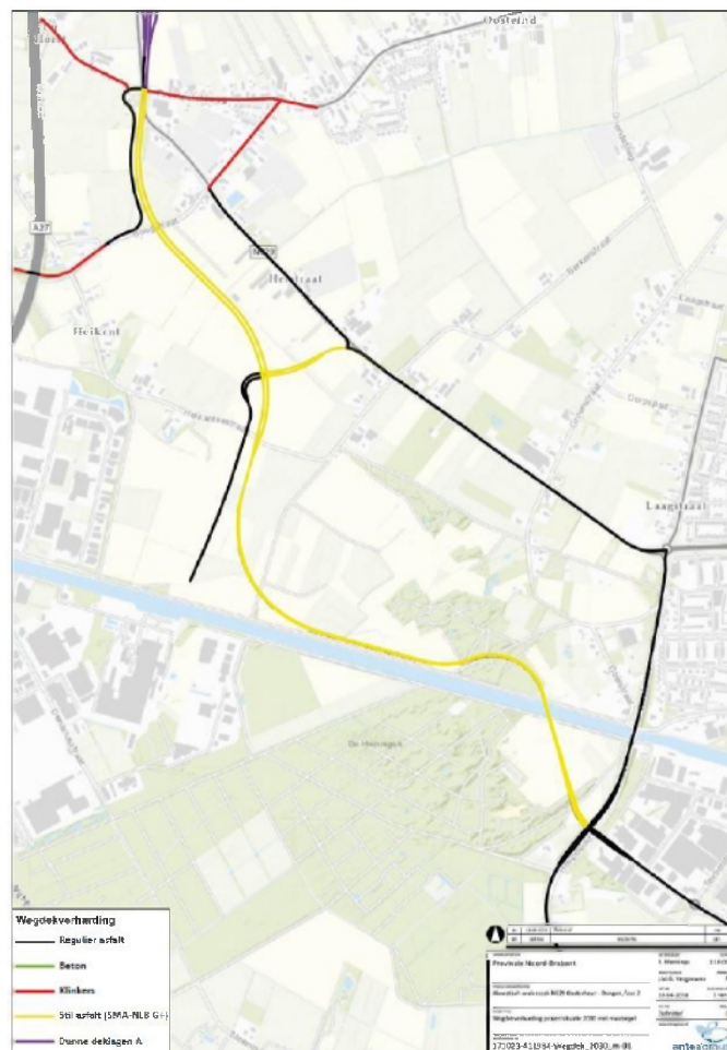
Figuur 6.1 Wegdekverhardingen in de toekomstige situatie van de N629.
