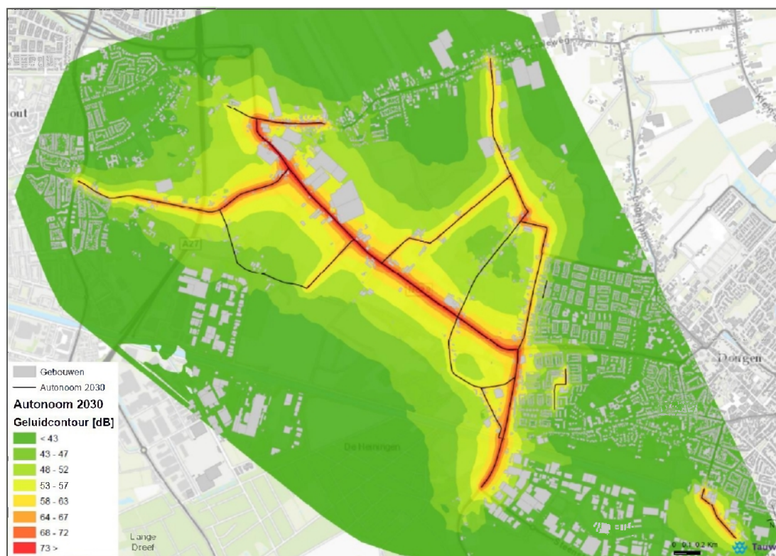
Figuur 1 Weergave geluidcontouren Lden referentie (autonome situatie, 2030)
