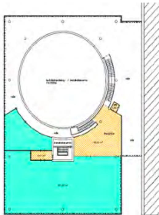
Eerste verdieping STC-gebouw (400 m 2 )
