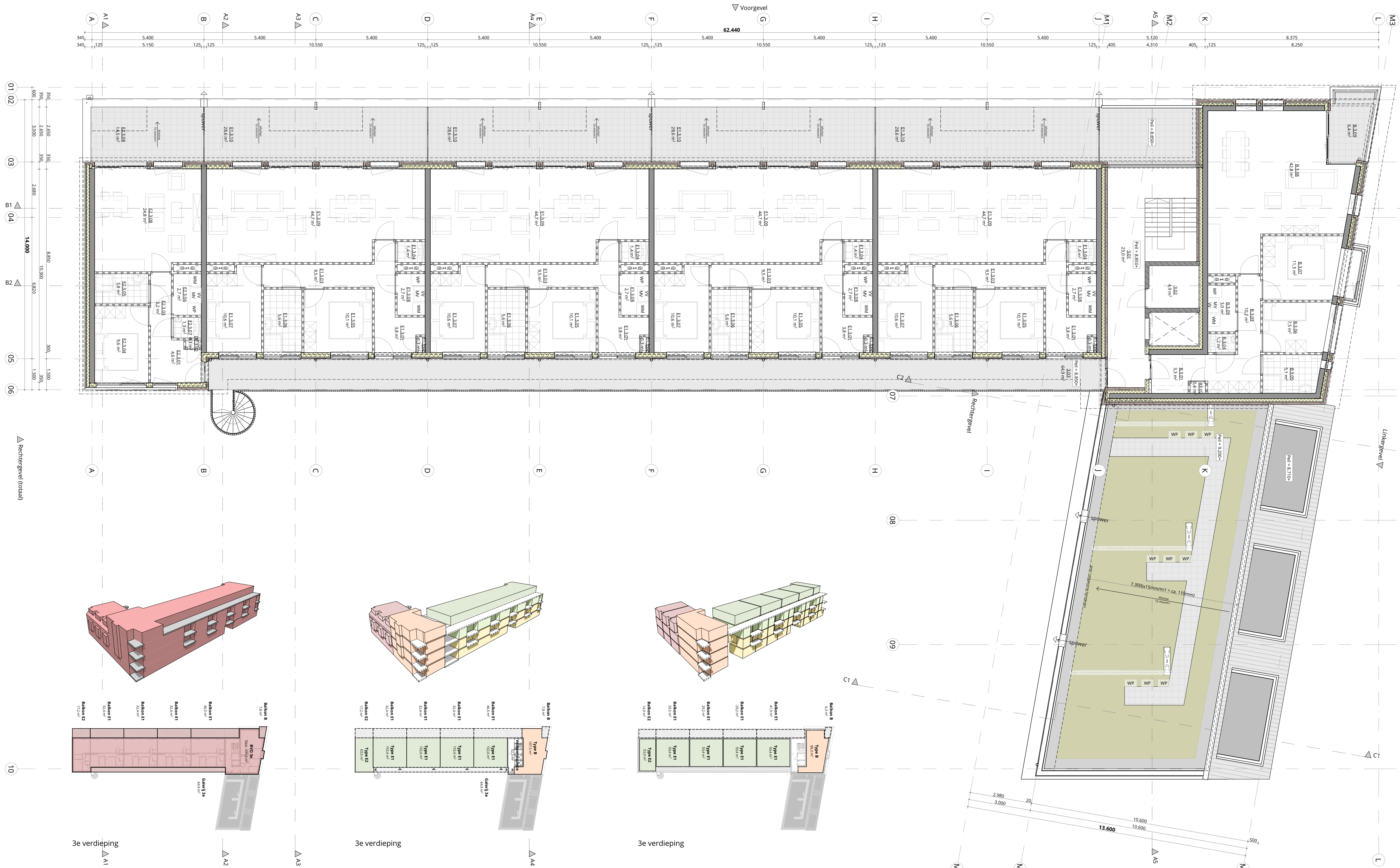
3e verdieping Schaal 1:100
